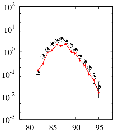
^{208}\text{Pb}(p,x)\text{Sr}
