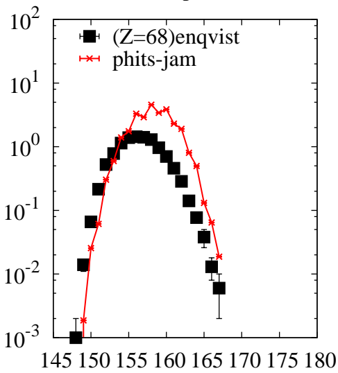
^{208}\text{Pb}(p,x)\text{Er}
