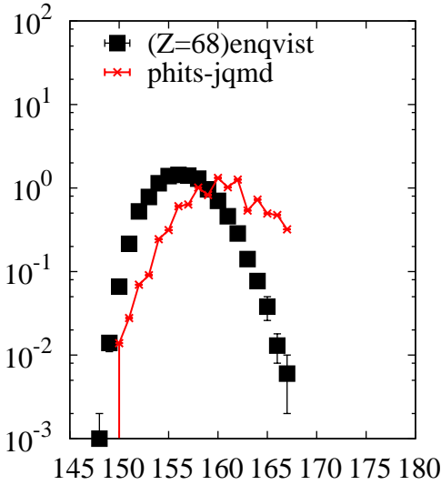
^{208}\text{Pb}(p,x)\text{Er}
