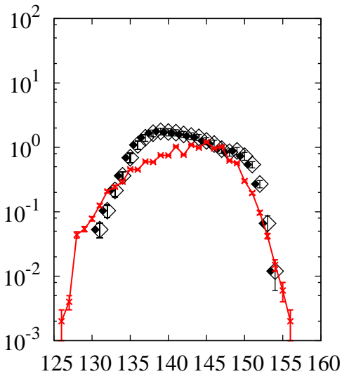
^{238}\text{U}(p,x)\text{Pr}
