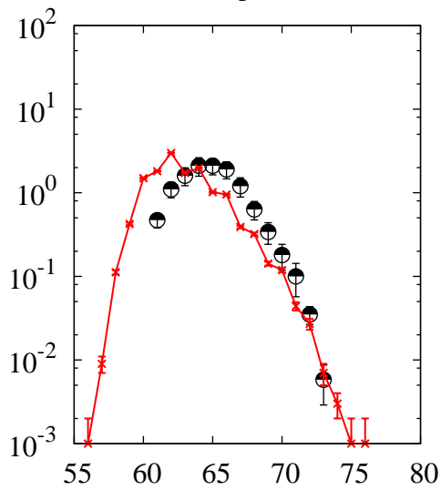
^{238}\text{U}(p,x)\text{Ni}
