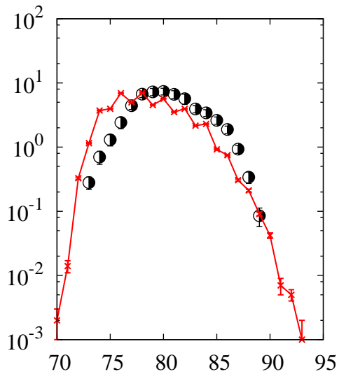
^{238}\text{U}(p,x)\text{Se}
