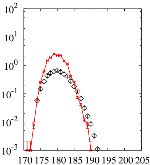
^{238}\text{U}(p,x)\text{Ir}
