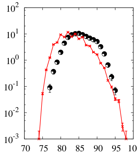
^{238}\text{U}(p,x)\text{Kr}
