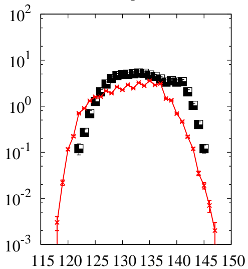
^{238}\text{U}(p,x)\text{Cs}
