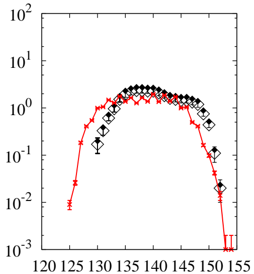
^{238}\text{U}(p,x)\text{Ce}
