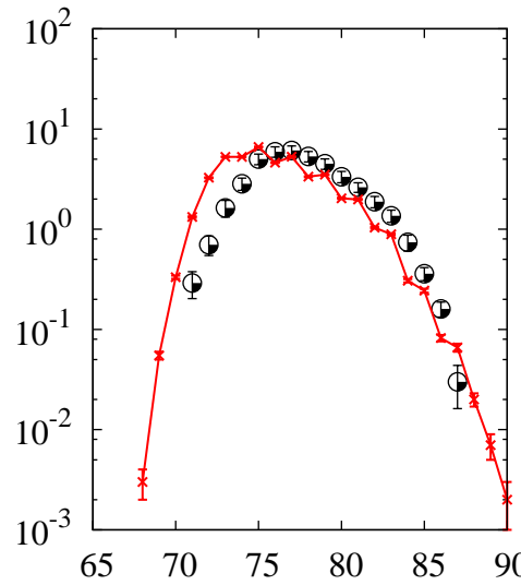
^{238}\text{U}(p,x)\text{As}
