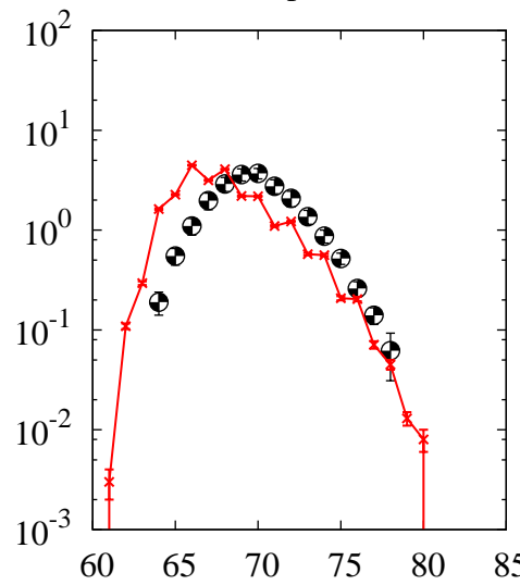
^{238}\text{U}(p,x)\text{Zn}
