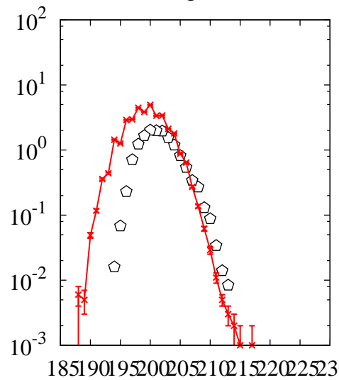
^{238}\text{U}(p,x)\text{Po}
