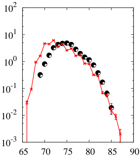
^{238}\text{U}(p,x)\text{Ge}
