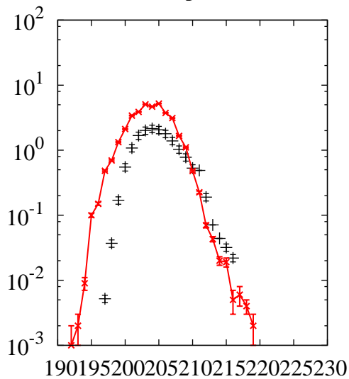
^{238}\text{U}(p,x)\text{At}
