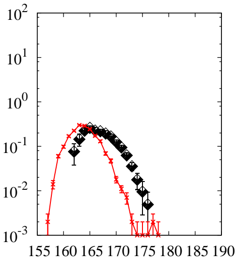
^{238}\text{U}(p,x)\text{Lu}
