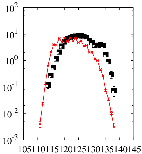
^{238}\text{U}(p,x)\text{Te}
