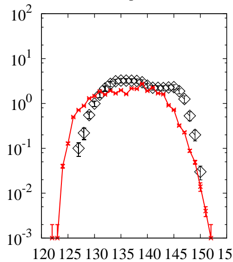
^{238}\text{U}(p,x)\text{La}
