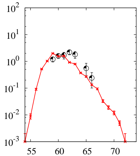
^{238}\text{U}(p,x)\text{Co}
