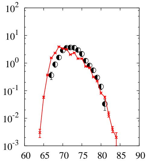
^{238}\text{U}(p,x)\text{Ga}
