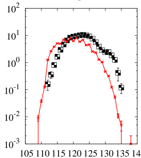
^{238}\text{U}(p,x)\text{Sb}
