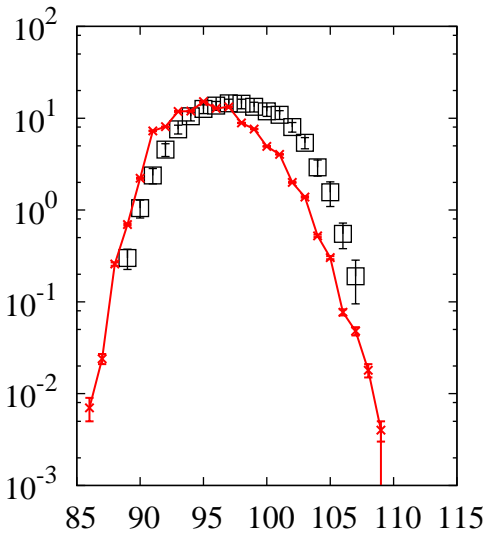
^{238}\text{U}(p,x)\text{Nb}
