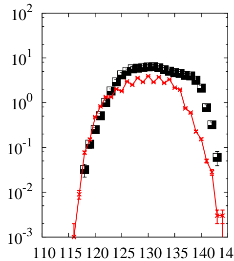
^{238}\text{U}(p,x)\text{Xe}
