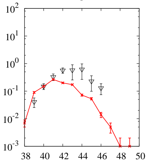
^{238}\text{U}(p,x)\text{K}
