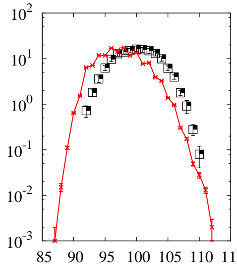
^{238}\text{U}(p,x)\text{Mo}
