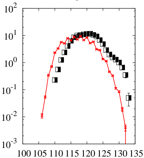
^{238}\text{U}(p,x)\text{Sn}
