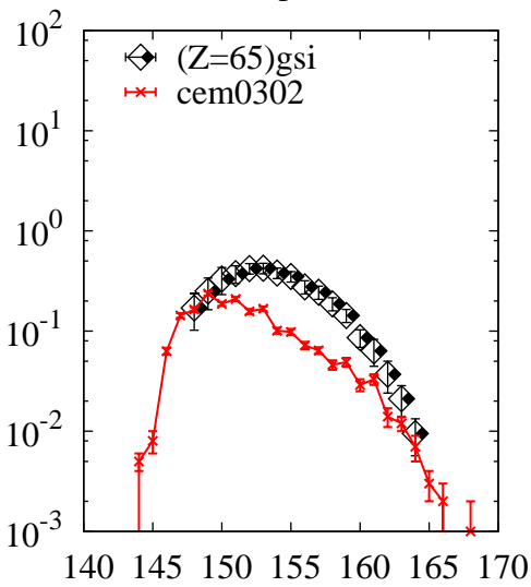
^{238}\text{U}(p,x)\text{Tb}
