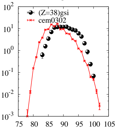
^{238}\text{U}(p,x)\text{Sr}
