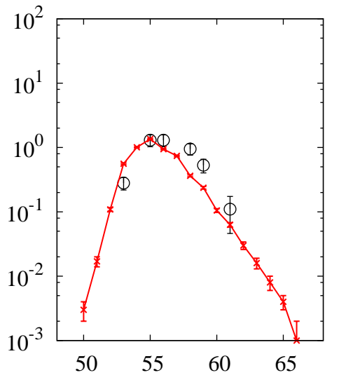
^{238}\text{U}(p,x)\text{Mn}
