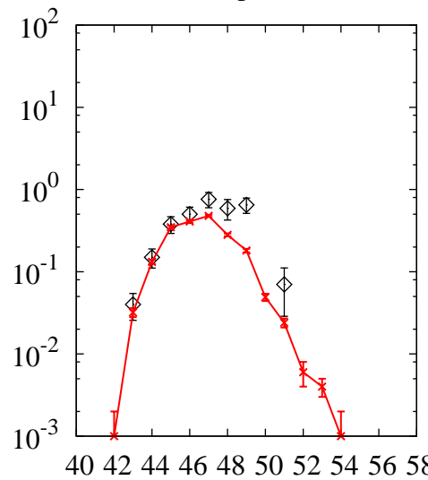
^{238}\text{U}(p,x)\text{Sc}
