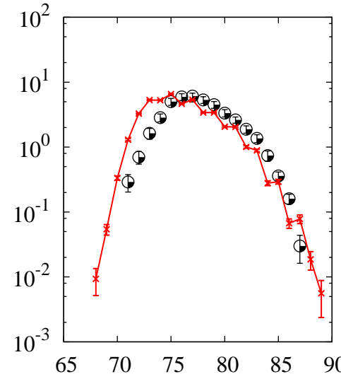
^{238}\text{U}(p,x)\text{As}
