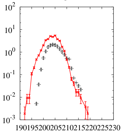
^{238}\text{U}(p,x)\text{At}
