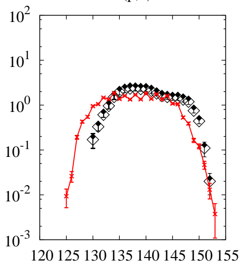
^{238}\text{U}(p,x)\text{Ce}
