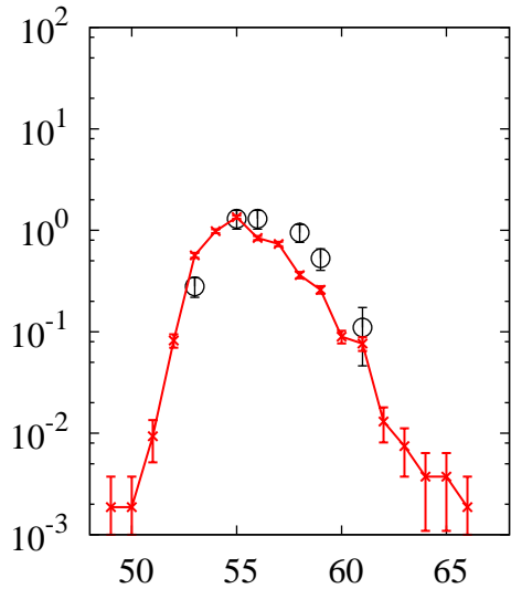
^{238}\text{U}(p,x)\text{Mn}
