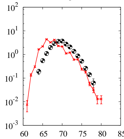
^{238}\text{U}(p,x)\text{Zn}
