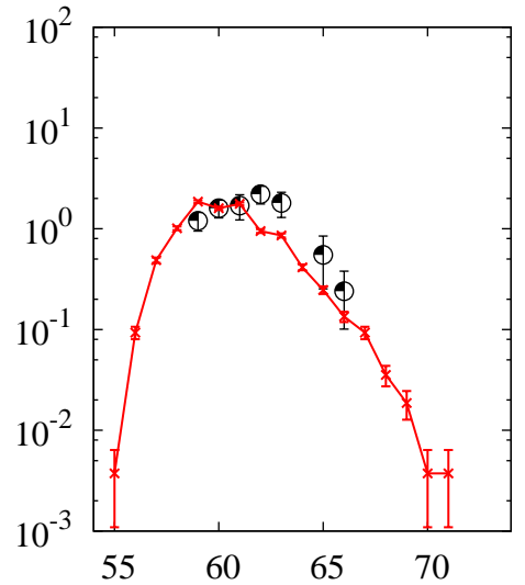
^{238}\text{U}(p,x)\text{Co}
