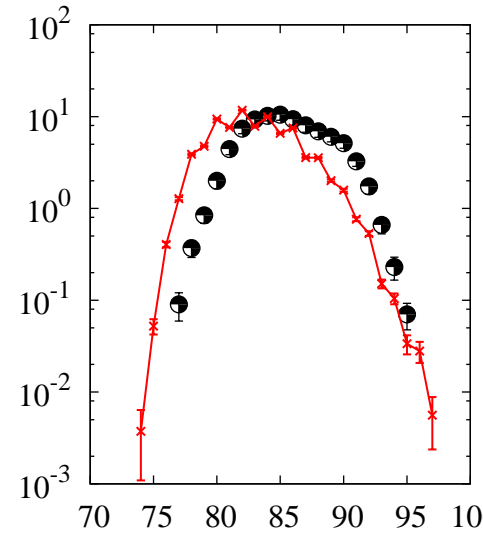
^{238}\text{U}(p,x)\text{Kr}
