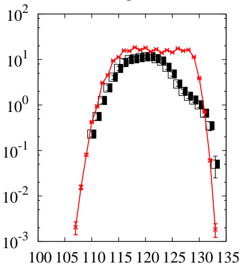
^{238}\text{U}(p,x)\text{Sn}
