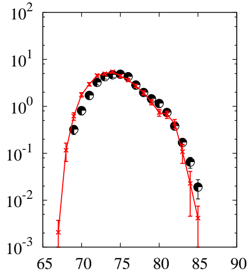
^{238}\text{U}(p,x)\text{Ge}
