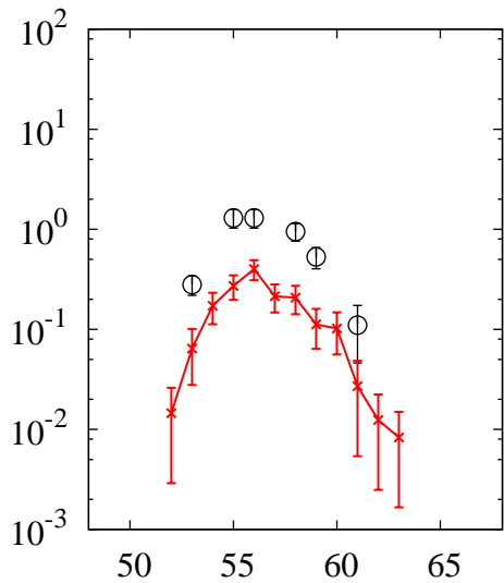
^{238}\text{U}(p,x)\text{Mn}
