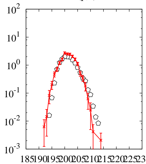
^{238}\text{U}(p,x)\text{Po}
