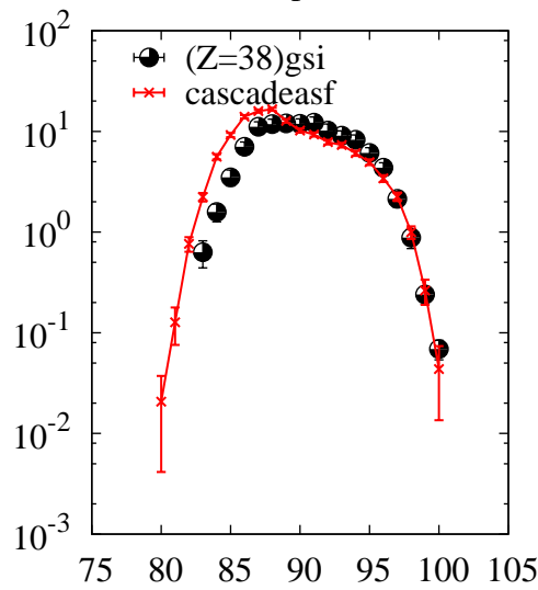
^{238}\text{U}(p,x)\text{Sr}
