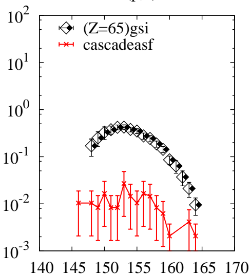
^{238}\text{U}(p,x)\text{Tb}
