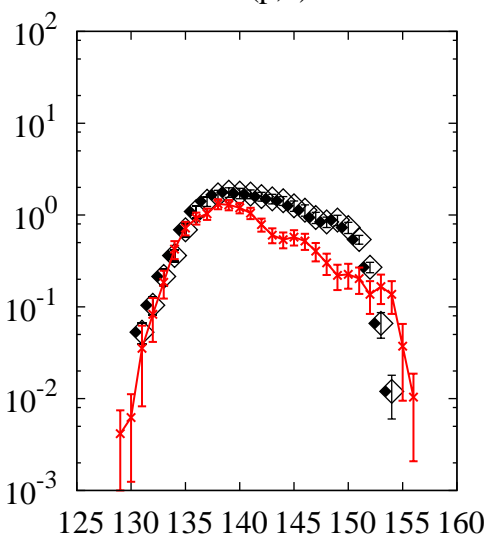
^{238}\text{U}(p,x)\text{Pr}
