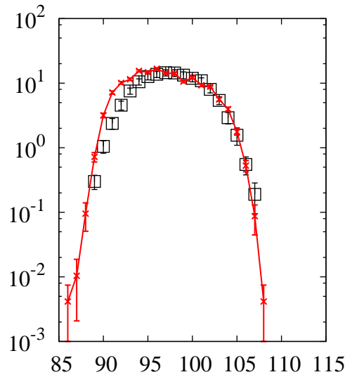
^{238}\text{U}(p,x)\text{Nb}
