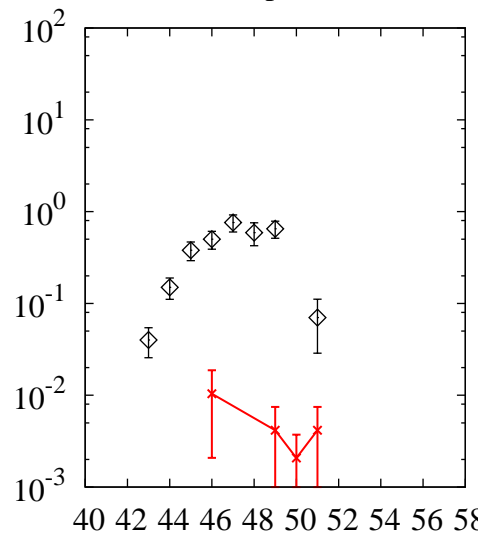
^{238}\text{U}(p,x)\text{Sc}
