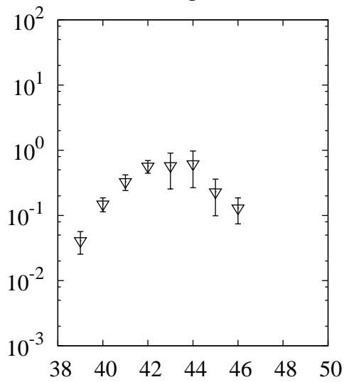
^{238}\text{U}(p,x)\text{K}
