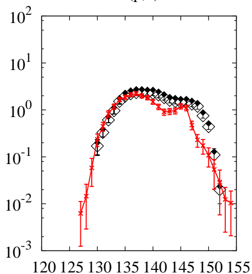
^{238}\text{U}(p,x)\text{Ce}
