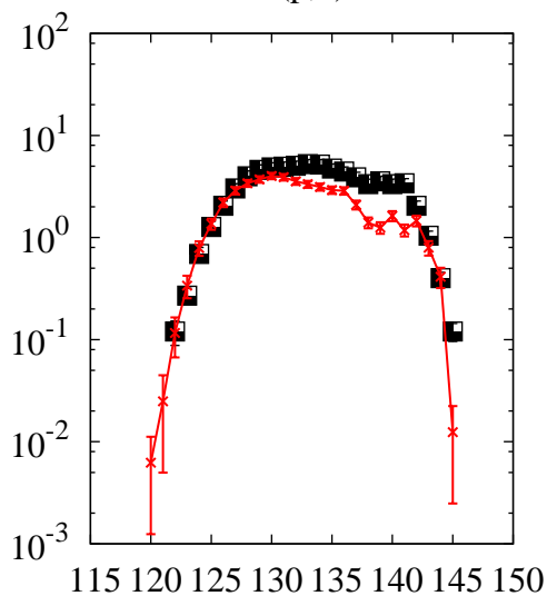
^{238}\text{U}(p,x)\text{Cs}
