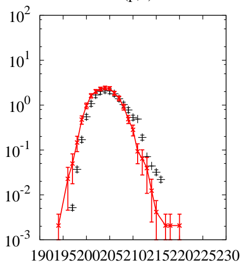
^{238}\text{U}(p,x)\text{At}
