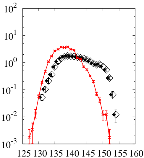
^{238}\text{U}(p,x)\text{Pr}
