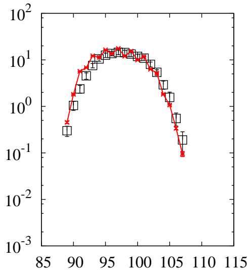
^{238}\text{U}(p,x)\text{Nb}
