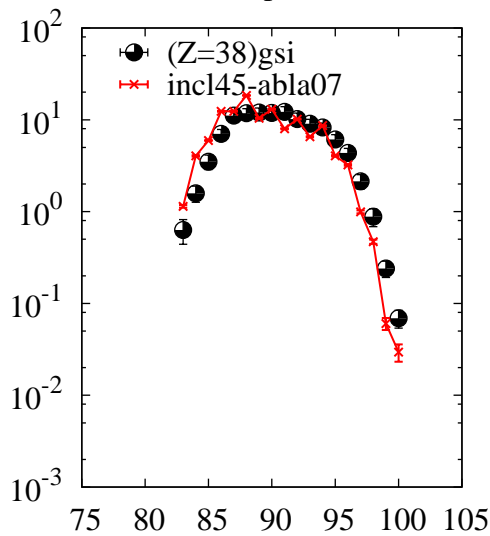
^{238}\text{U}(p,x)\text{Sr}
