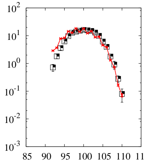
^{238}\text{U}(p,x)\text{Mo}
