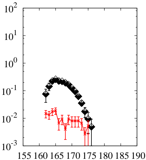
^{238}\text{U}(p,x)\text{Lu}
