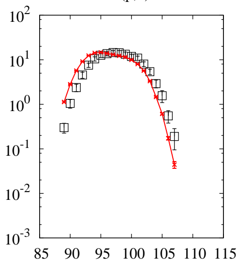
^{238}\text{U}(p,x)\text{Nb}
