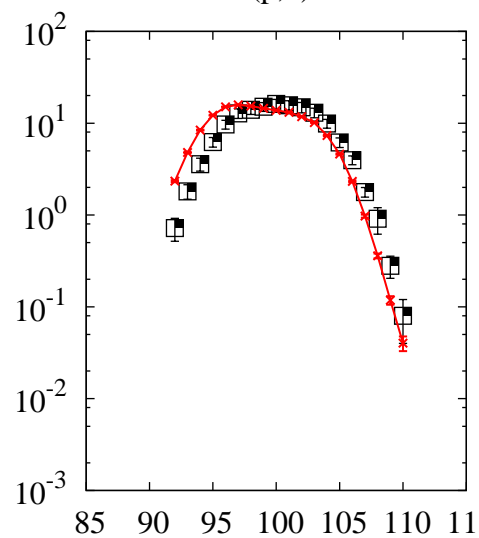
^{238}\text{U}(p,x)\text{Mo}
