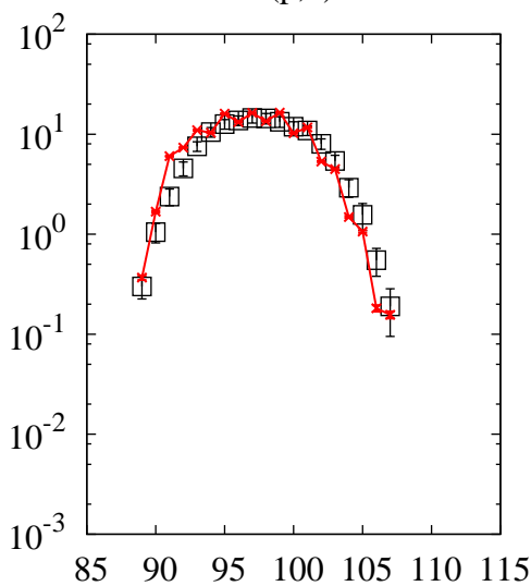
^{238}\text{U}(p,x)\text{Nb}
