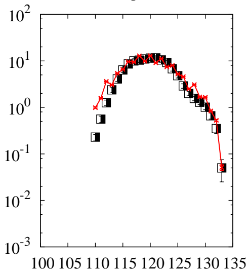
^{238}\text{U}(p,x)\text{Sn}
