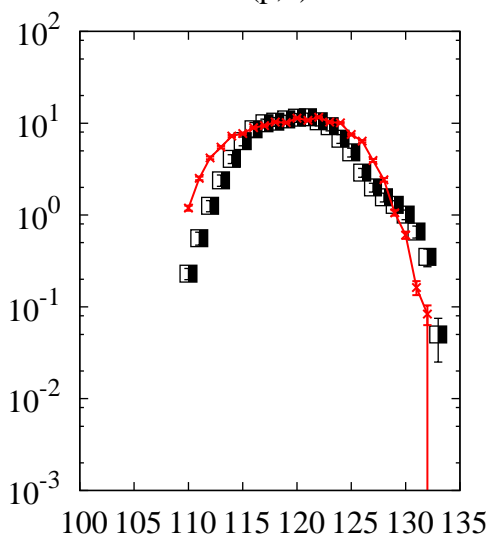
^{238}\text{U}(p,x)\text{Sn}
