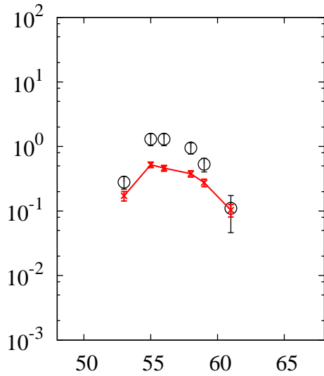
^{238}\text{U}(p,x)\text{Mn}
