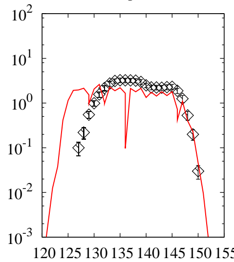
^{238}\text{U}(p,x)\text{La}
