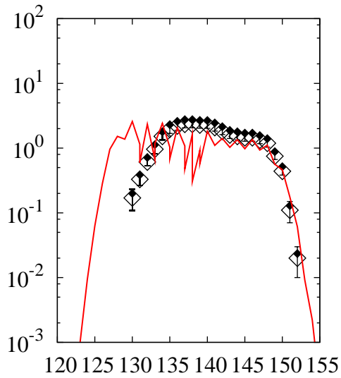
^{238}\text{U}(p,x)\text{Ce}
