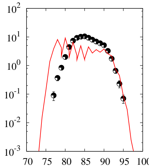
^{238}\text{U}(p,x)\text{Kr}
