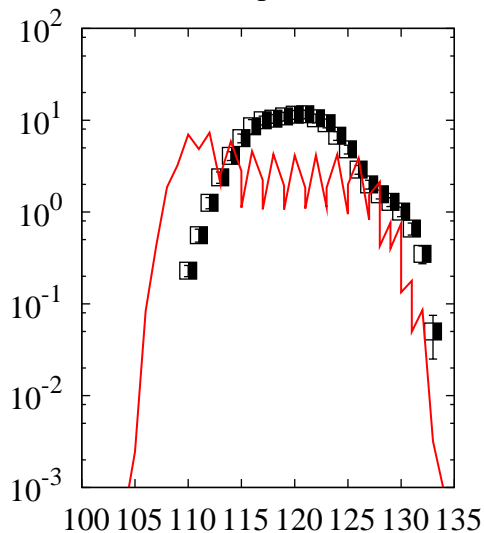
^{238}\text{U}(p,x)\text{Sn}
