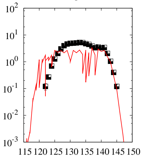
^{238}\text{U}(p,x)\text{Cs}
