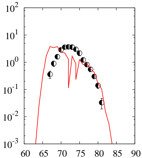
^{238}\text{U}(p,x)\text{Ga}
