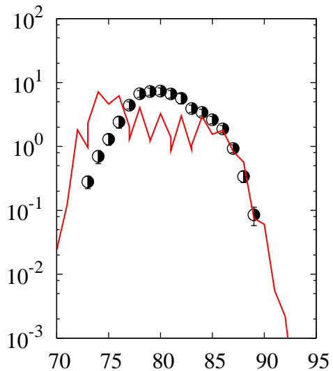
^{238}\text{U}(p,x)\text{Se}
