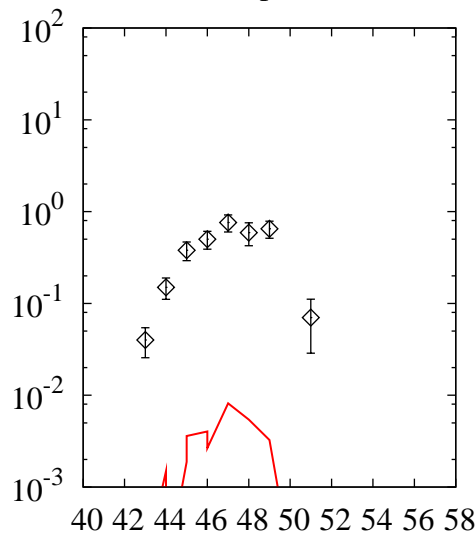
^{238}\text{U}(p,x)\text{Sc}
