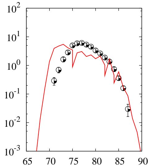
^{238}\text{U}(p,x)\text{As}
