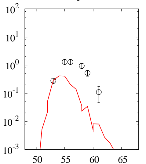
^{238}\text{U}(p,x)\text{Mn}
