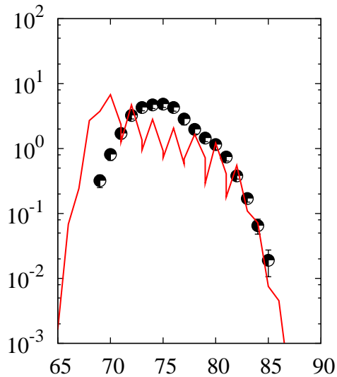
^{238}\text{U}(p,x)\text{Ge}
