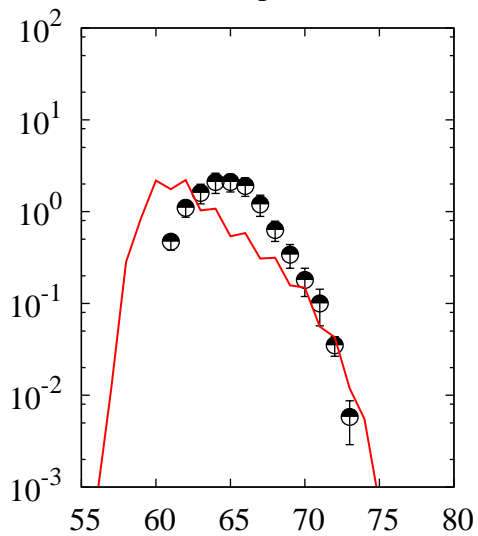
^{238}\text{U}(p,x)\text{Ni}
