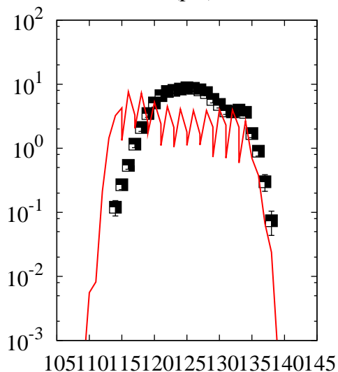
^{238}\text{U}(p,x)\text{Te}
