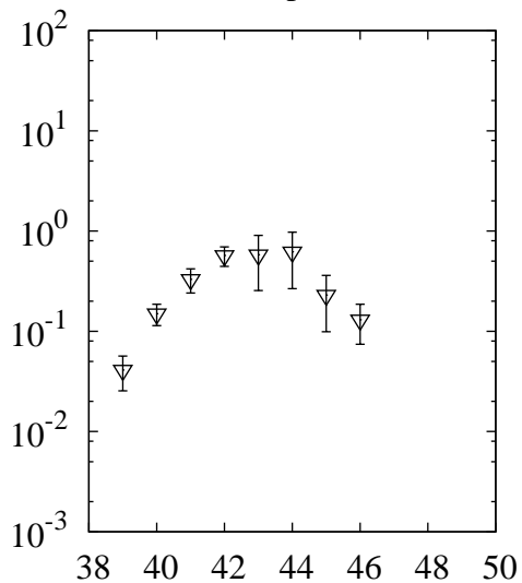
^{238}\text{U}(p,x)\text{K}
