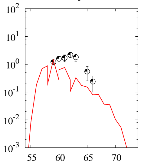
^{238}\text{U}(p,x)\text{Co}
