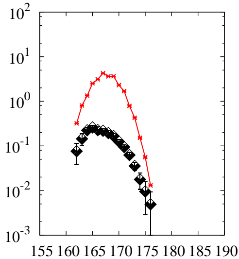
^{238}\text{U}(p,x)\text{Lu}
