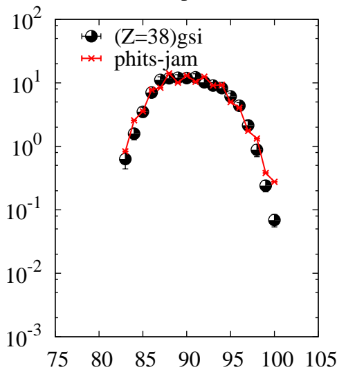
^{238}\text{U}(p,x)\text{Sr}
