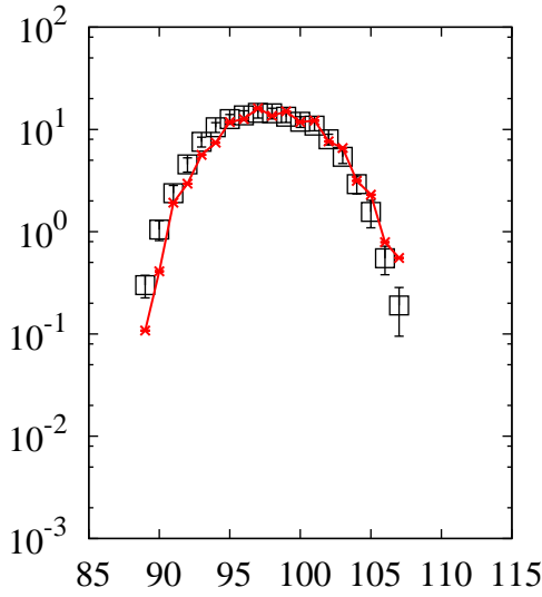
^{238}\text{U}(p,x)\text{Nb}
