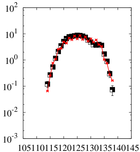
^{238}\text{U}(p,x)\text{Te}
