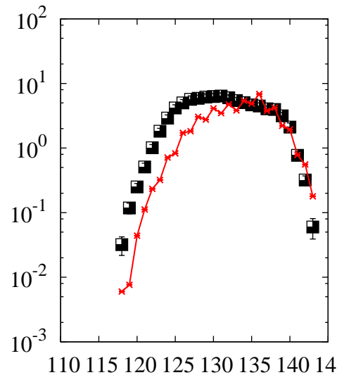
^{238}\text{U}(p,x)\text{Xe}
