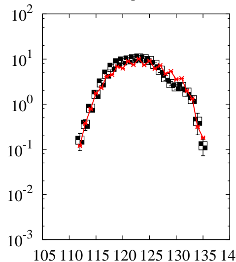
^{238}\text{U}(p,x)\text{Sb}
