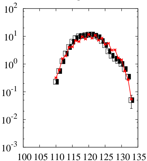
^{238}\text{U}(p,x)\text{Sn}
