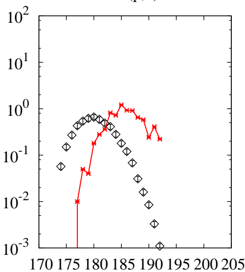
^{238}\text{U}(p,x)\text{Ir}
