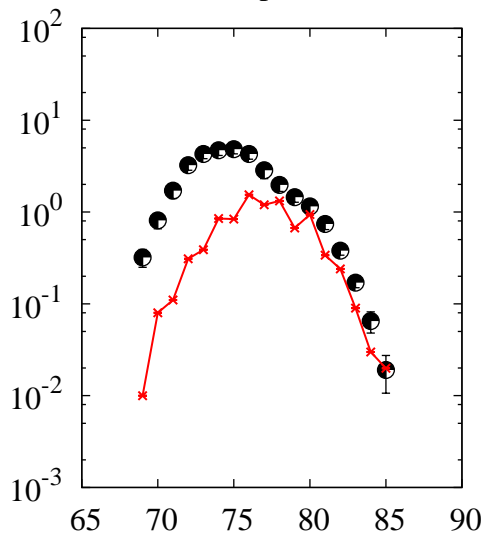
^{238}\text{U}(p,x)\text{Ge}
