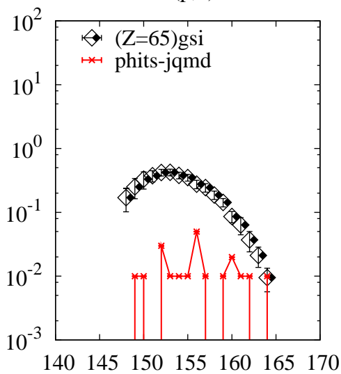
^{238}\text{U}(p,x)\text{Tb}
