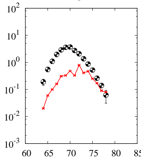
^{238}\text{U}(p,x)\text{Zn}
