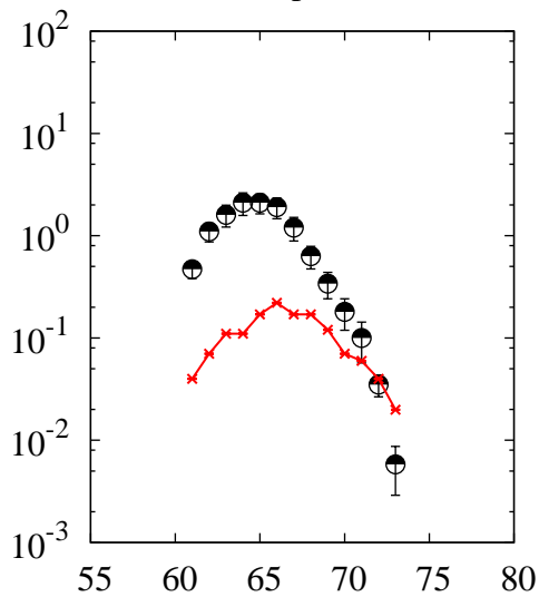
^{238}\text{U}(p,x)\text{Ni}
