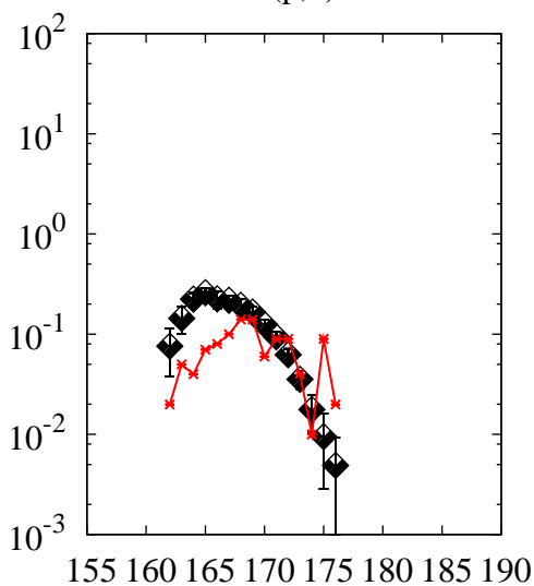
^{238}\text{U}(p,x)\text{Lu}
