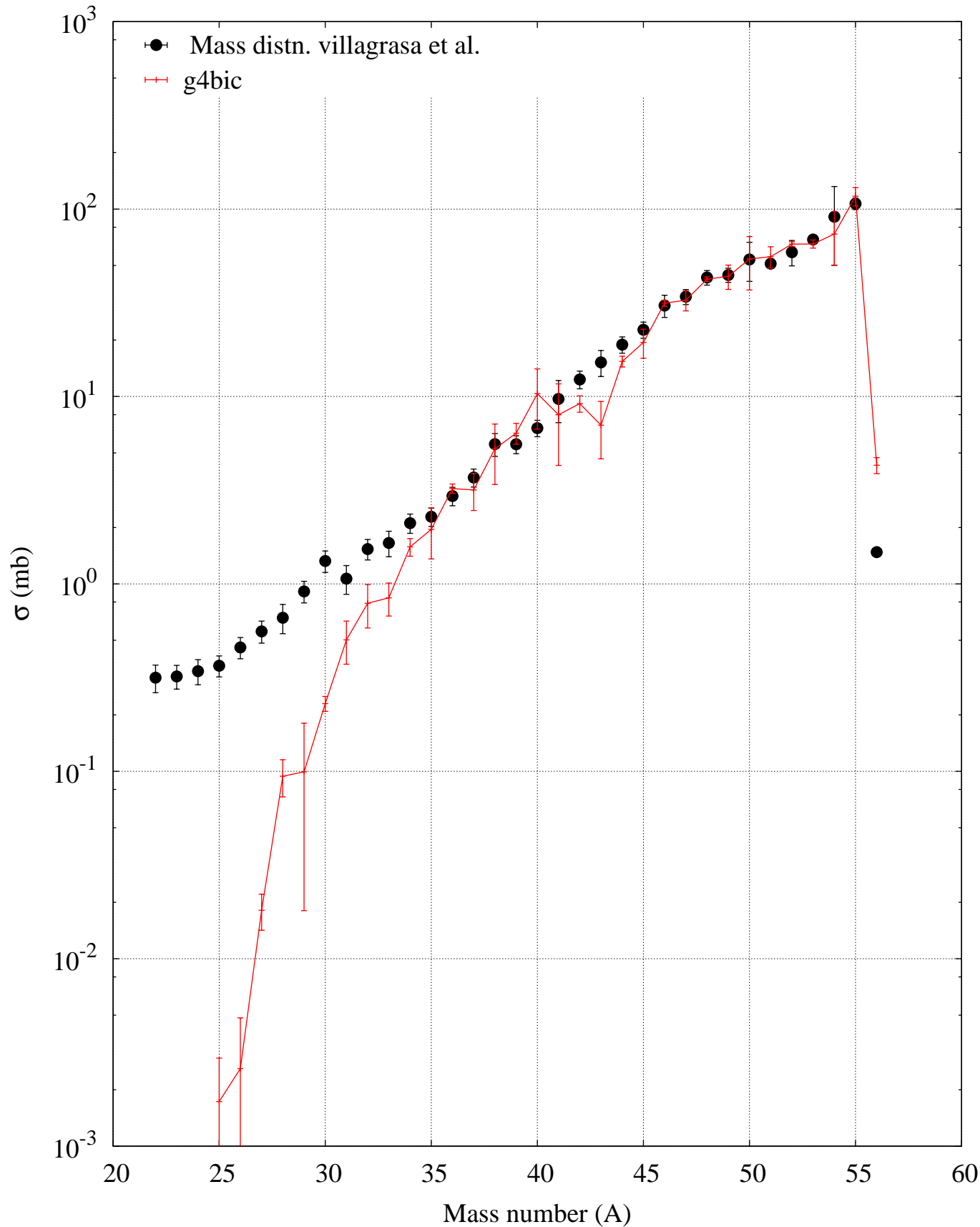
p (300 MeV) + Fe56 -- Residue mass production
