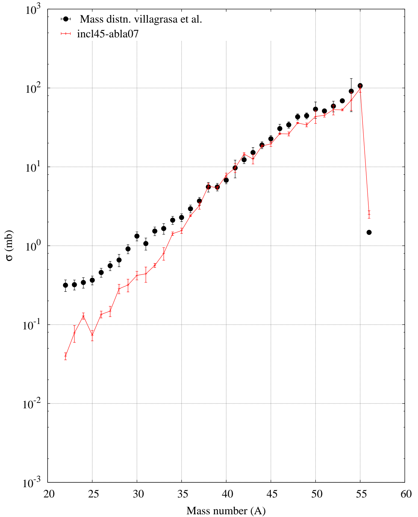
p (300 MeV) + Fe56 -- Residue mass production
