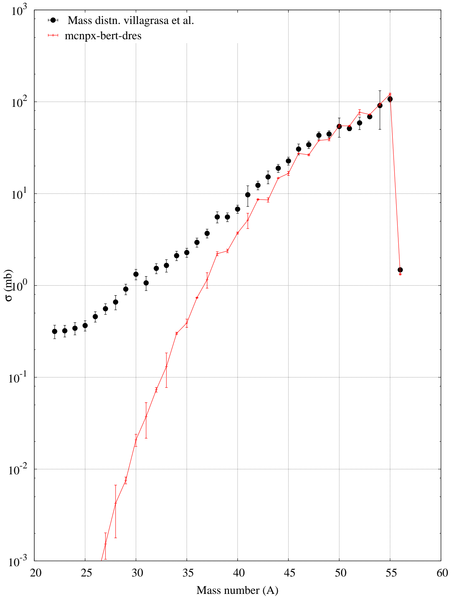
p (300 MeV) + Fe56 -- Residue mass production
