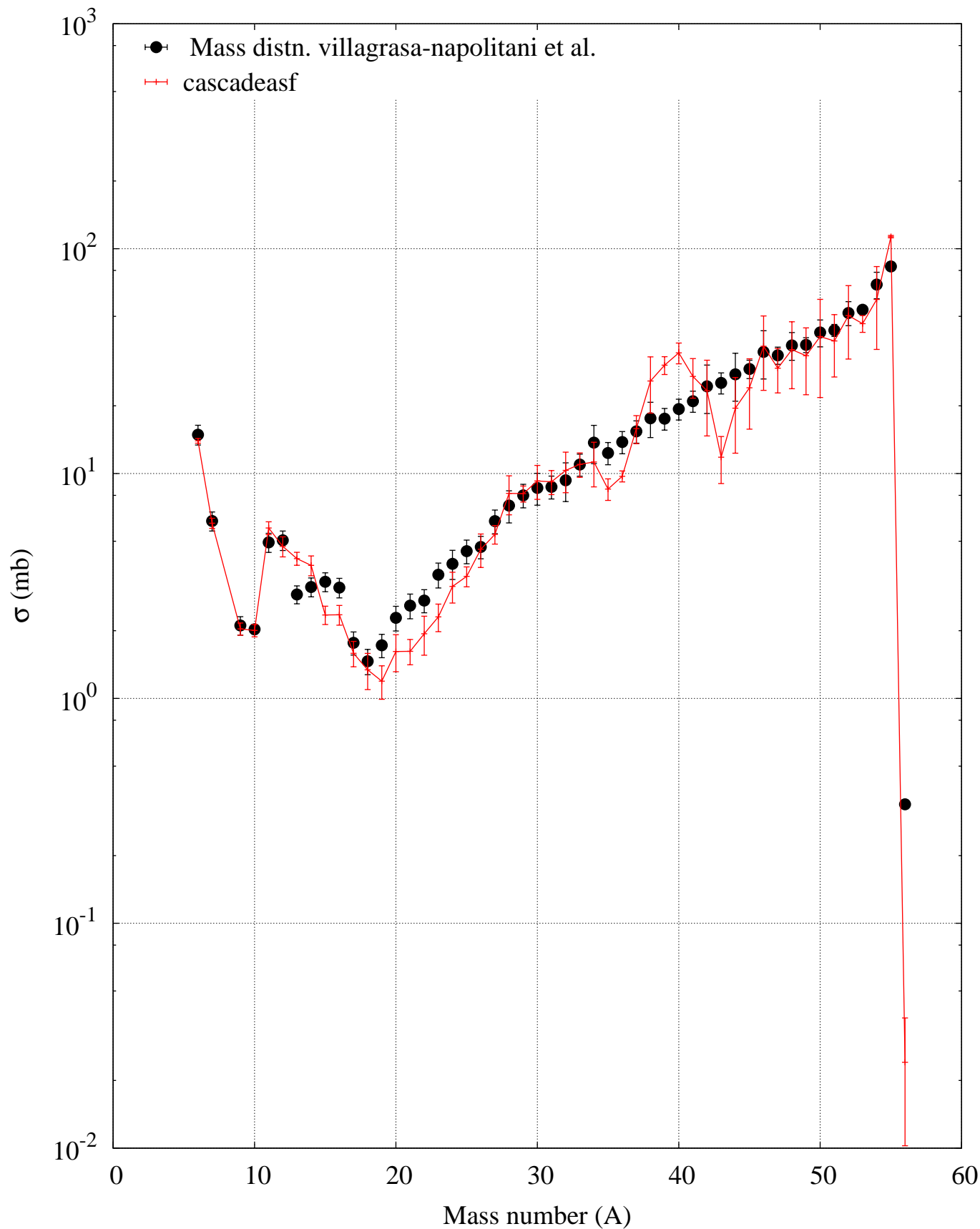
p (1000 MeV) + Fe56 -- Residue mass production
