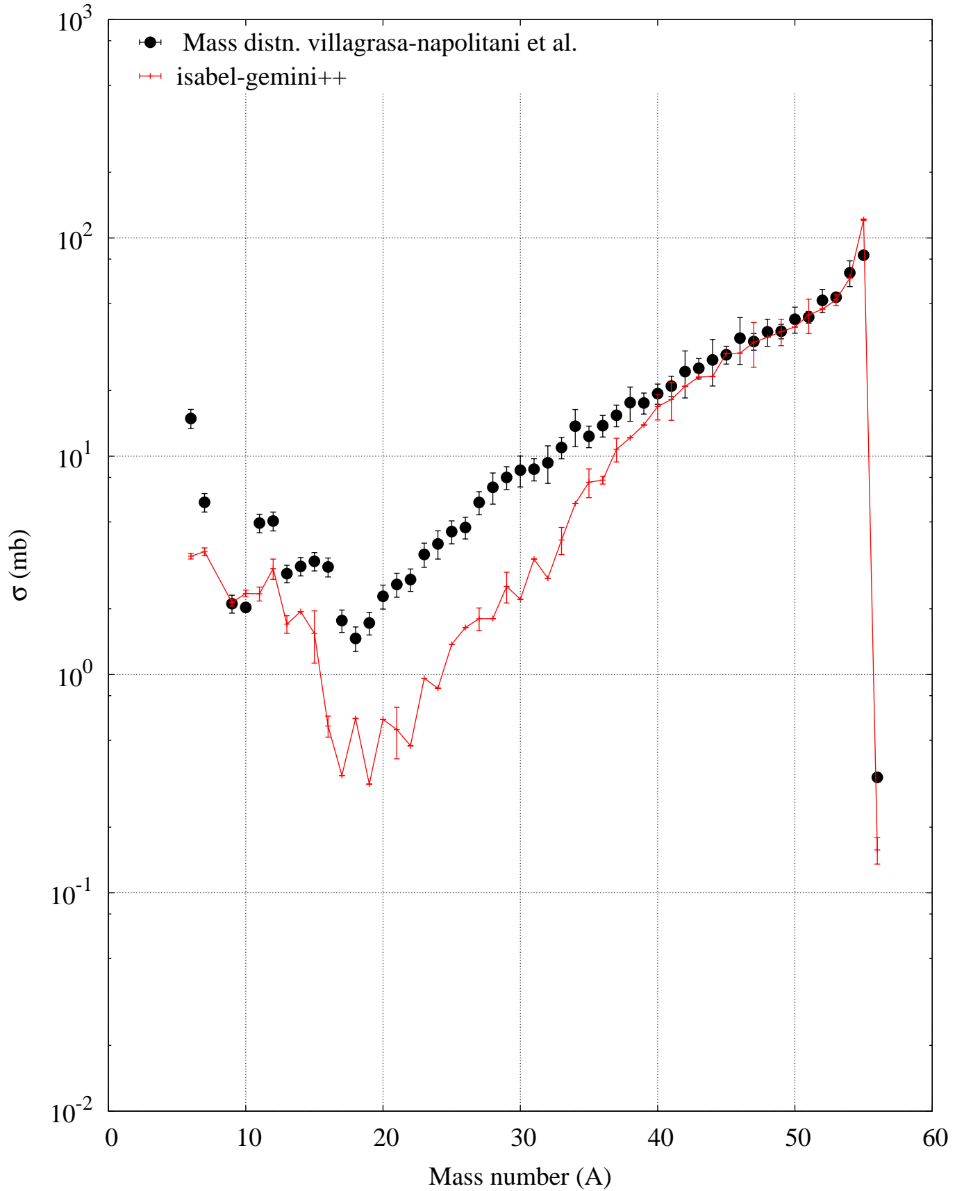
p (1000 MeV) + Fe56 -- Residue mass production
