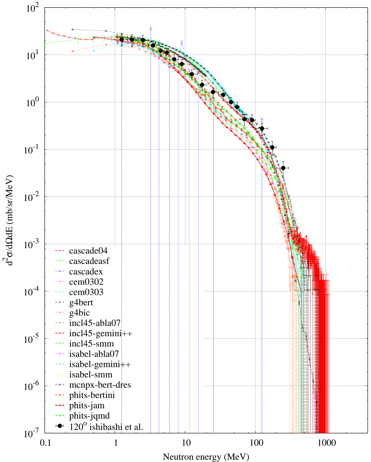
p (3000 MeV) + Fe -- Neutron spectrum
