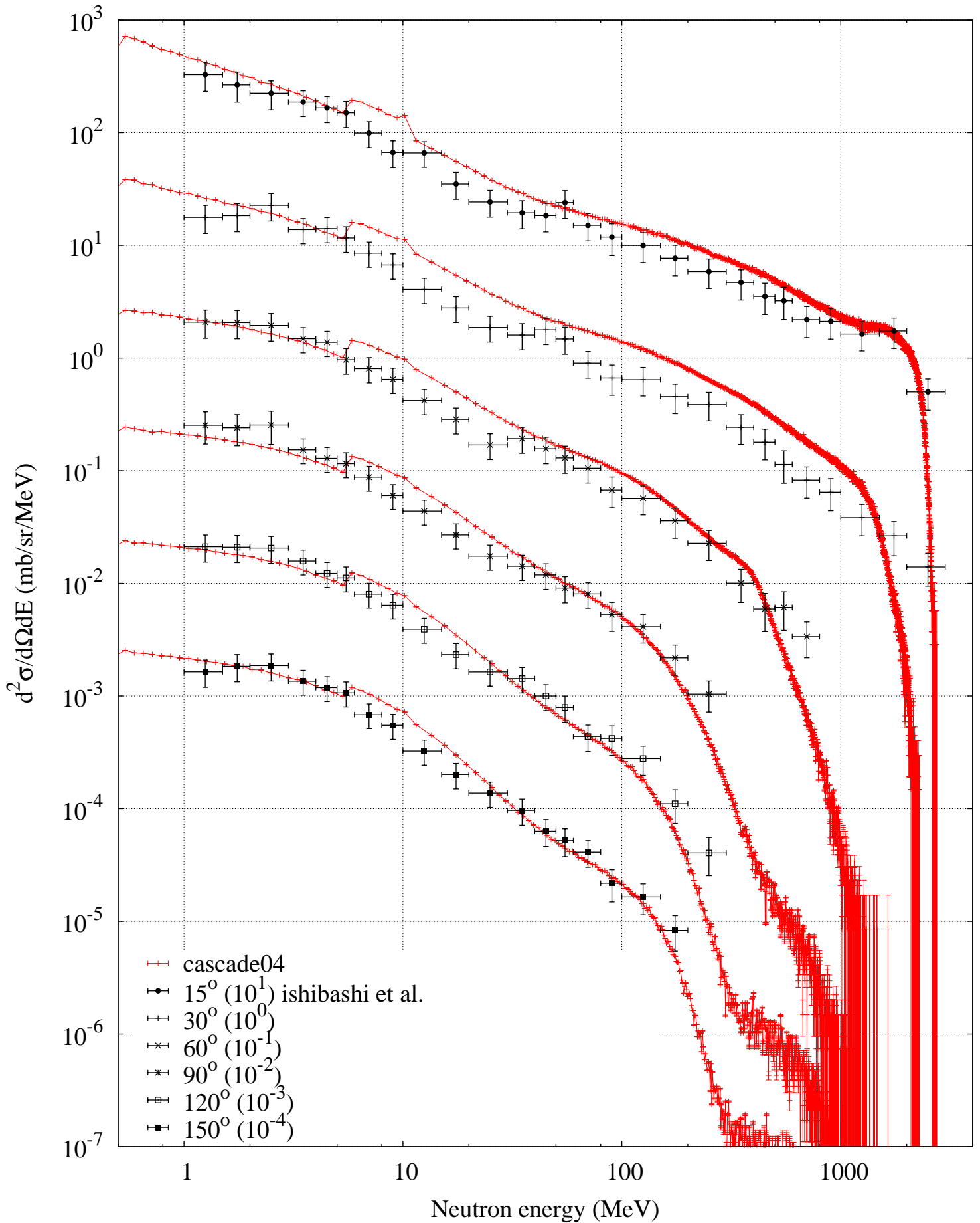
p (3000 MeV) + Fe -- Neutron spectrum
