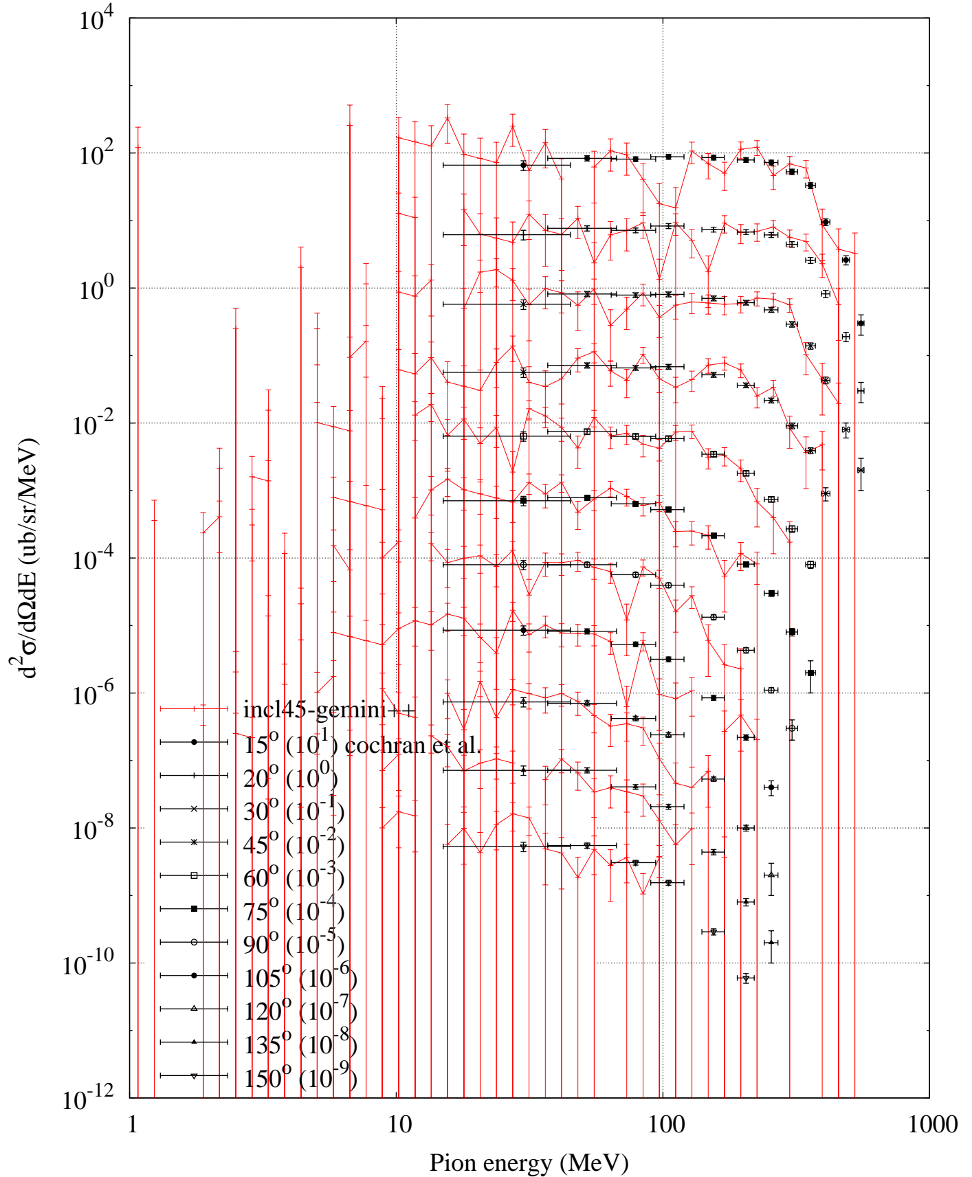
p (730 MeV) + Al -- Pion minus spectrum
