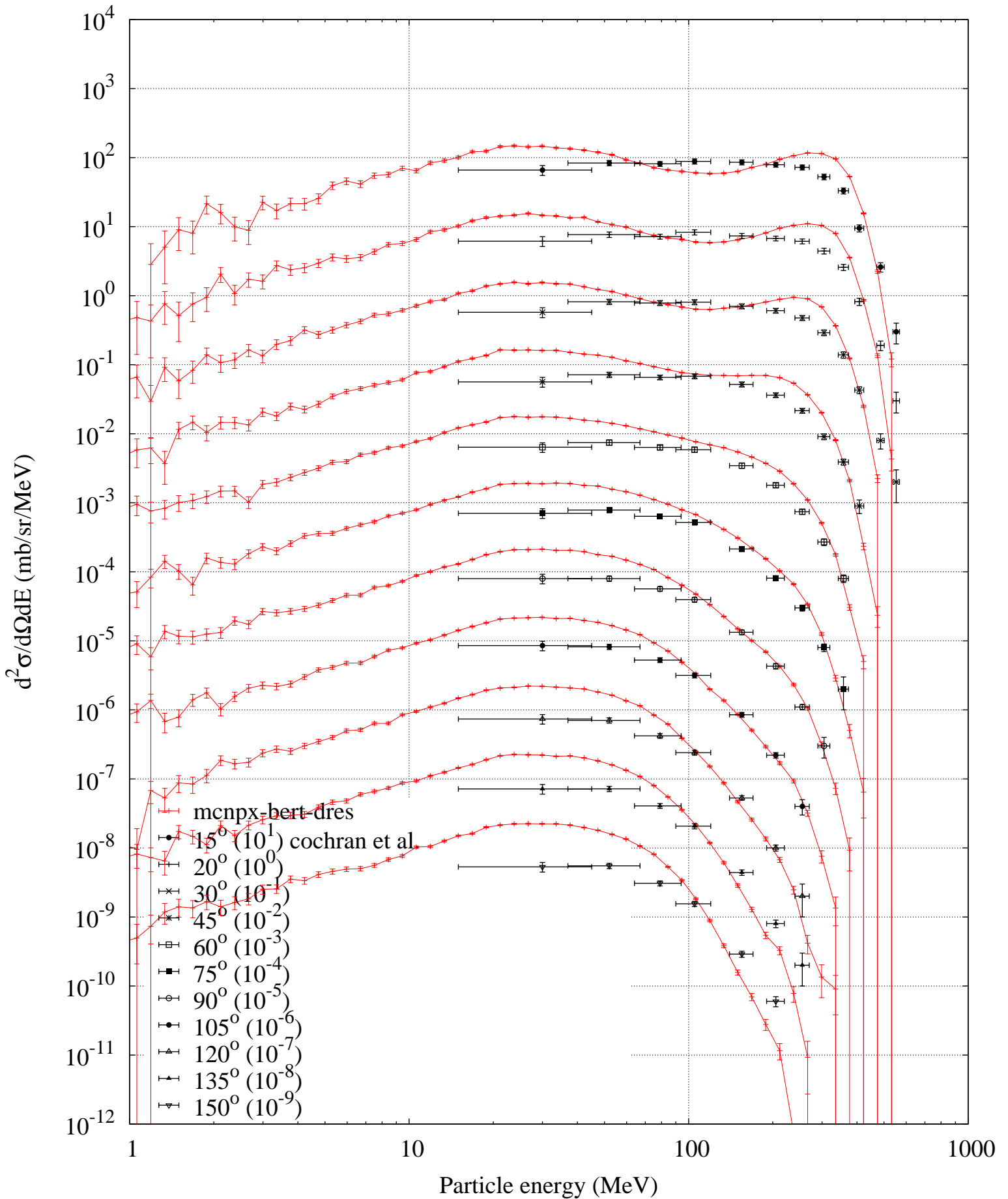
p (730 MeV) + Al -- Pion minus spectrum
