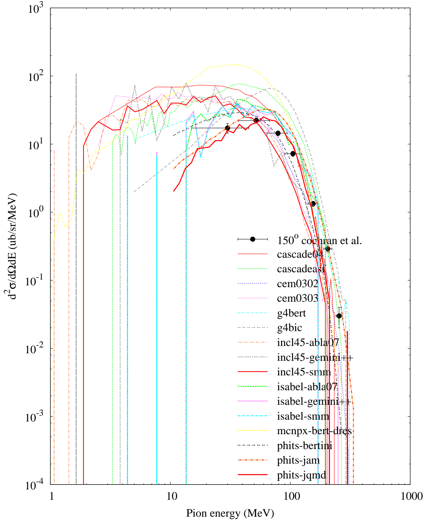
p (730 MeV) + Al --Pion plus spectrum
