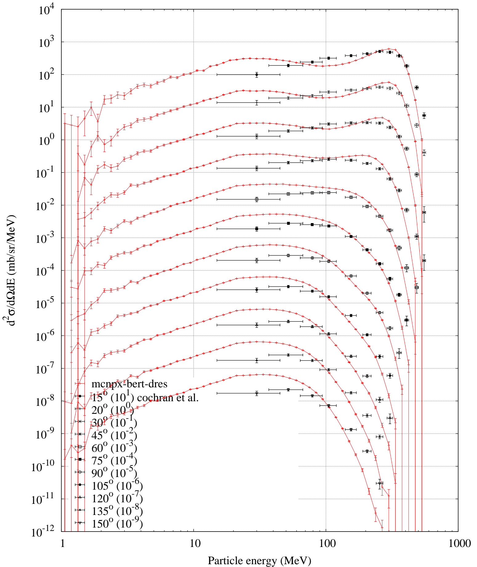
p (730 MeV) + Al -- Pion plus spectrum
