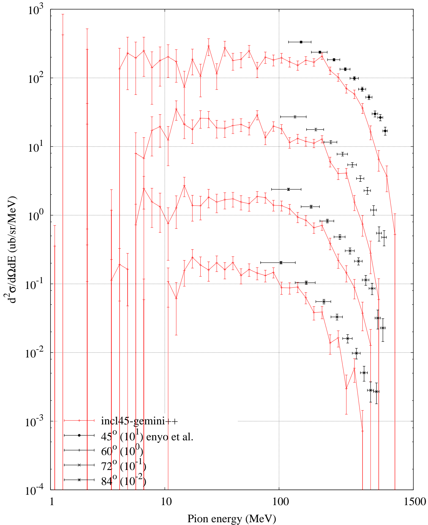
p (2205 MeV) + Al -- Pion minus spectrum
