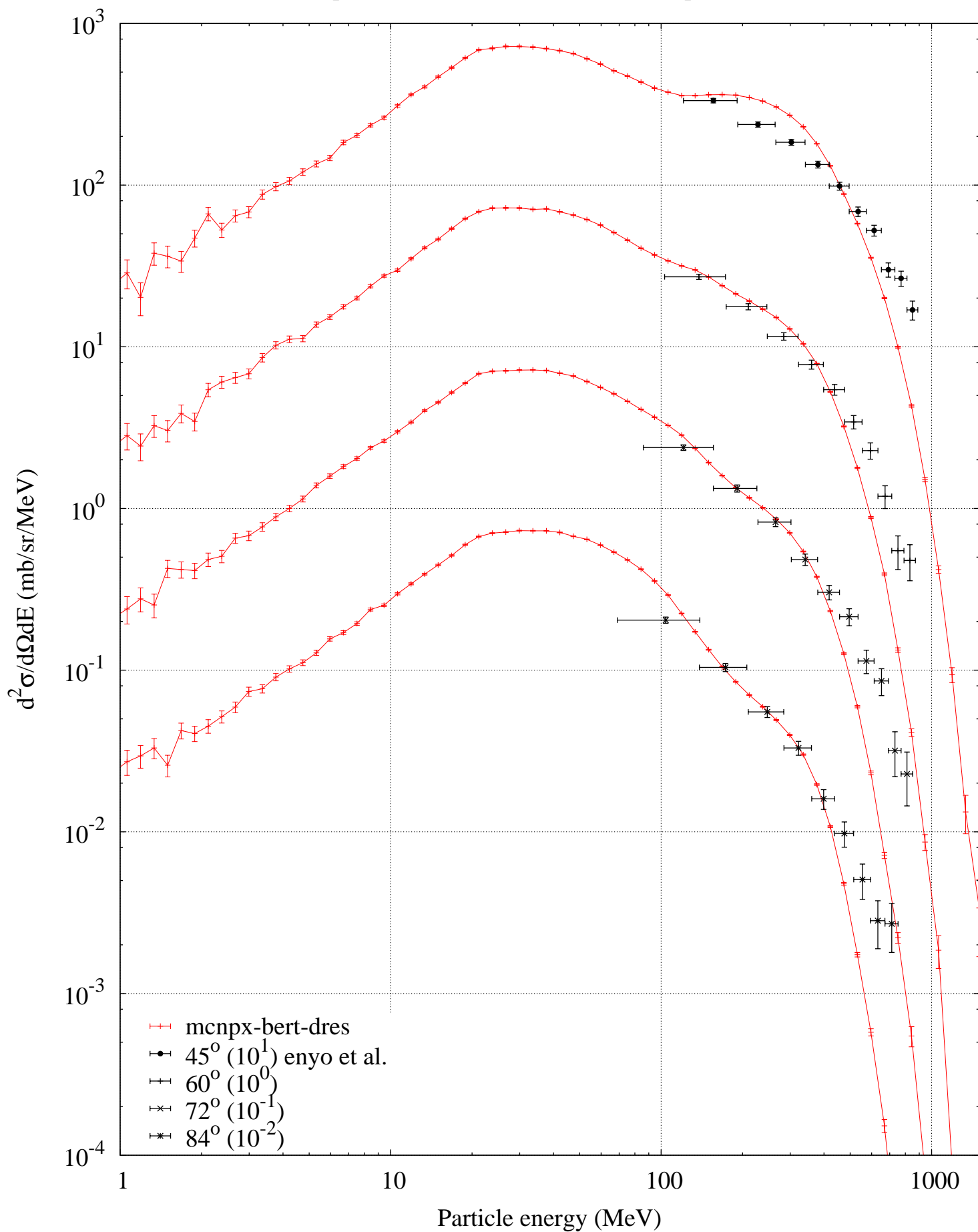
p (2205 MeV) + Al -- Pion minus spectrum
