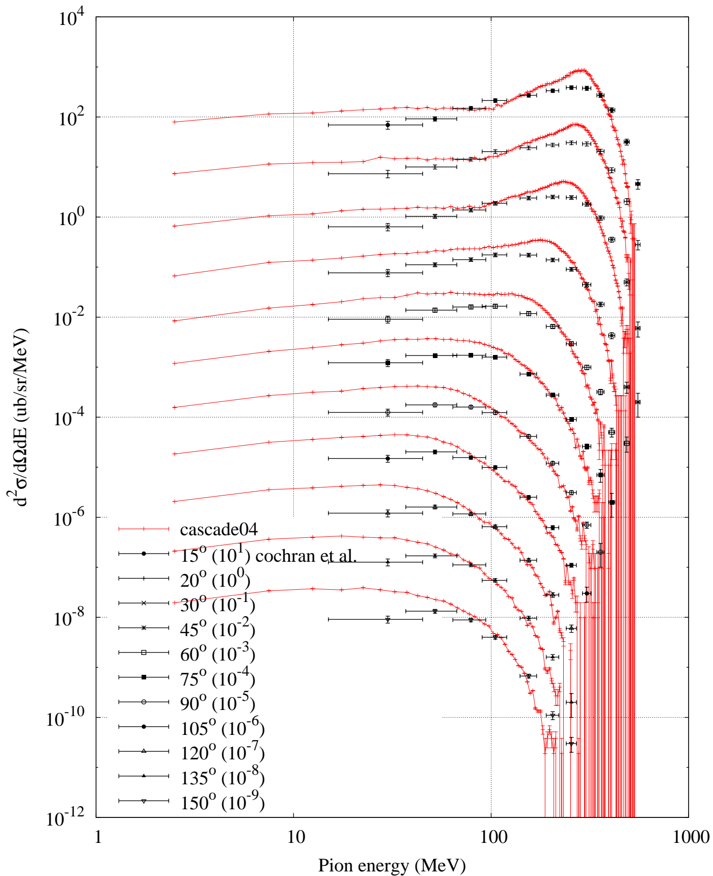
p (730 MeV) + C -- Pion plus spectrum
