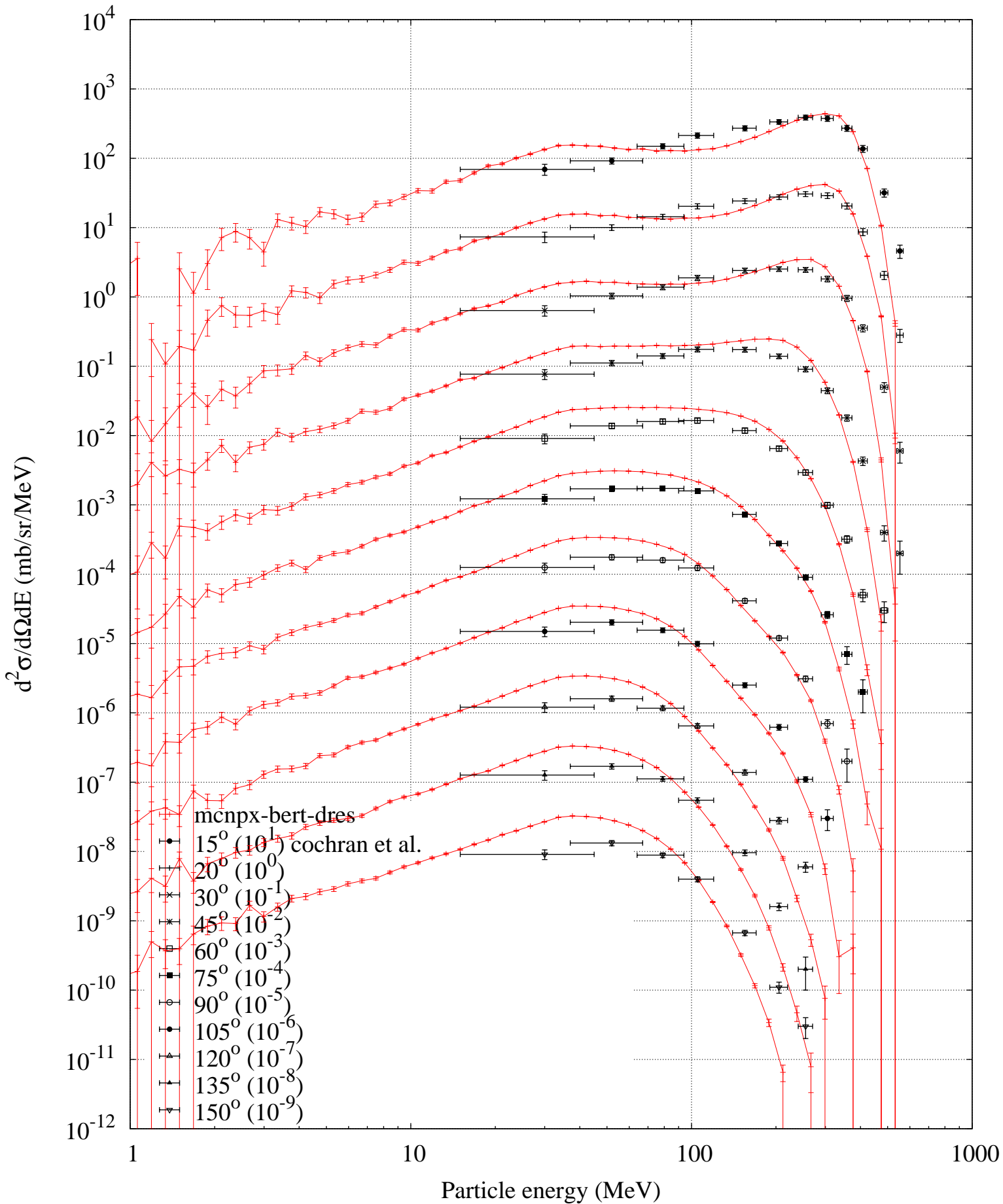
p (730 MeV) + C -- Pion plus spectrum
