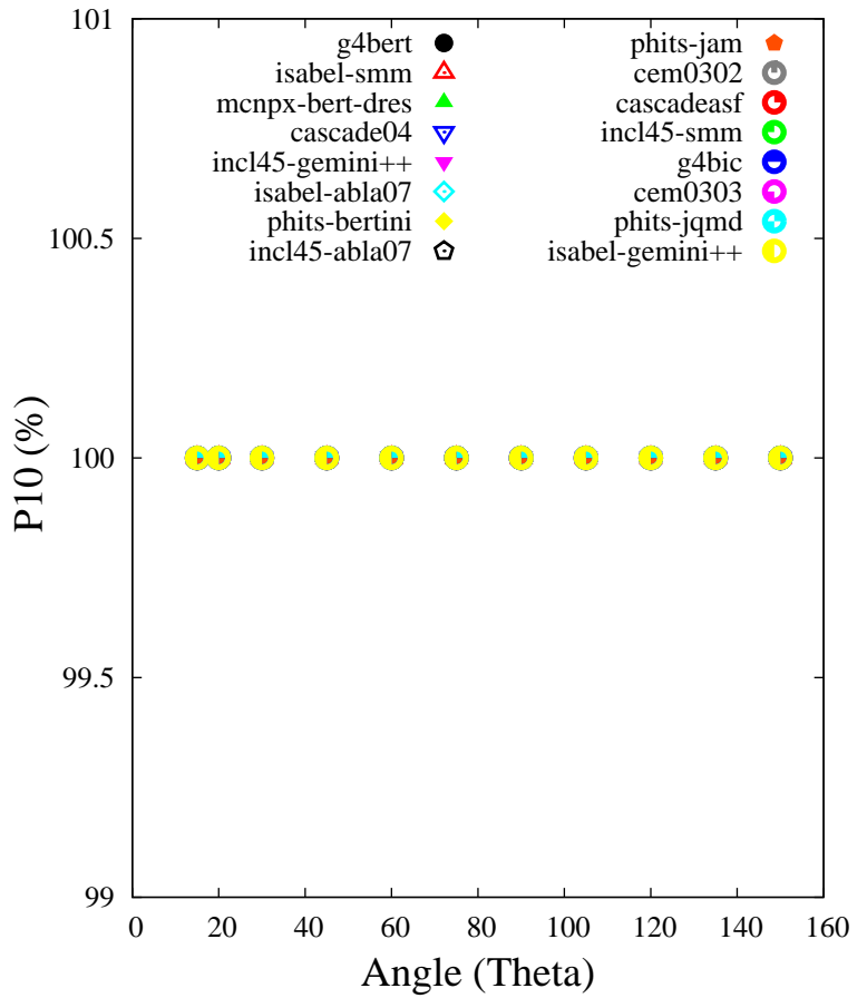
P10 factor - E_{int}(20-150 \text{ MeV})
