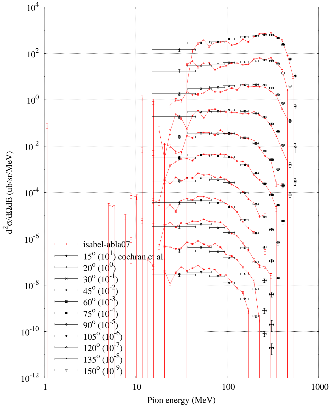
p (730 MeV) + Cu -- Pion plus spectrum
