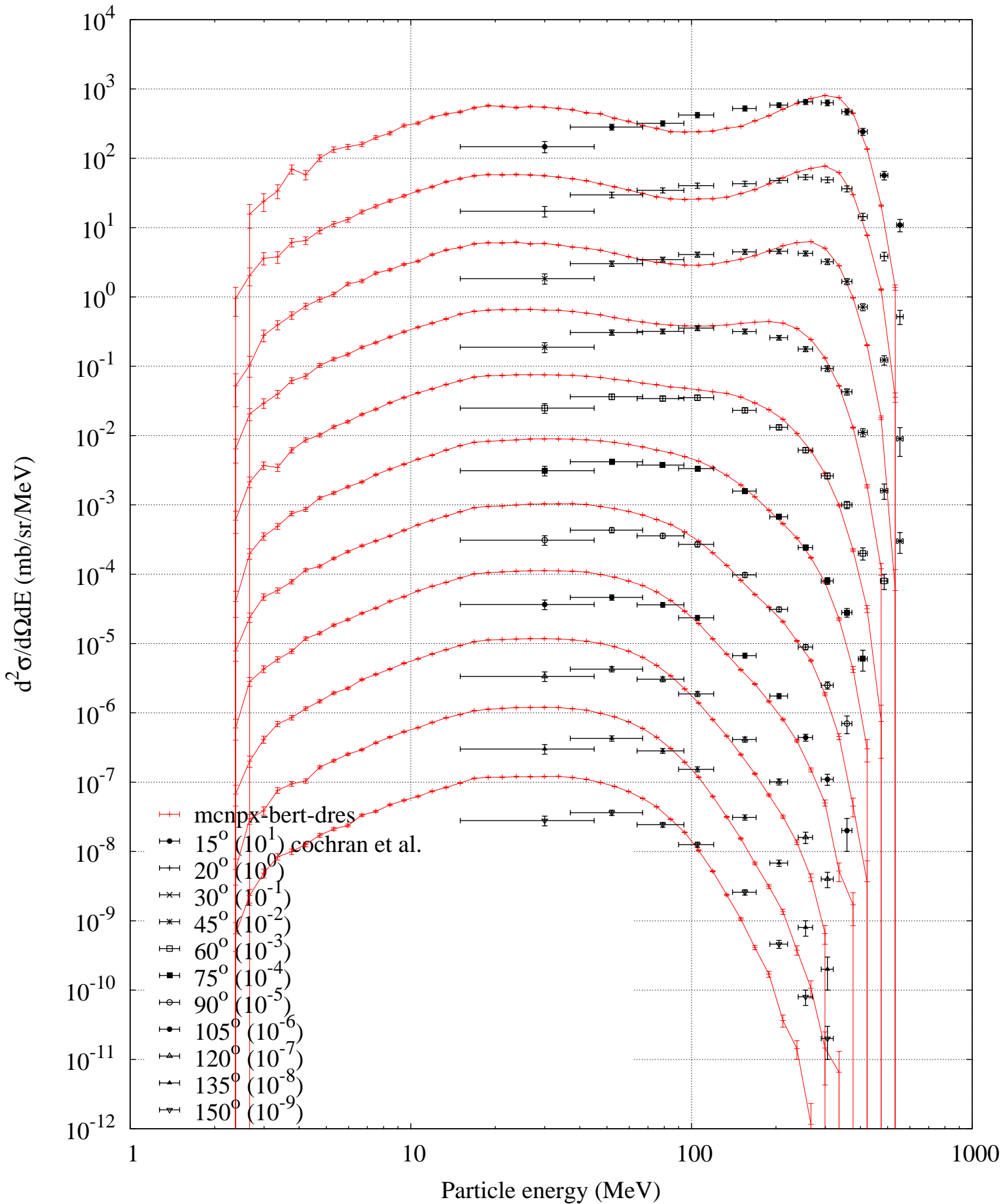
p (730 MeV) + Cu -- Pion plus spectrum
