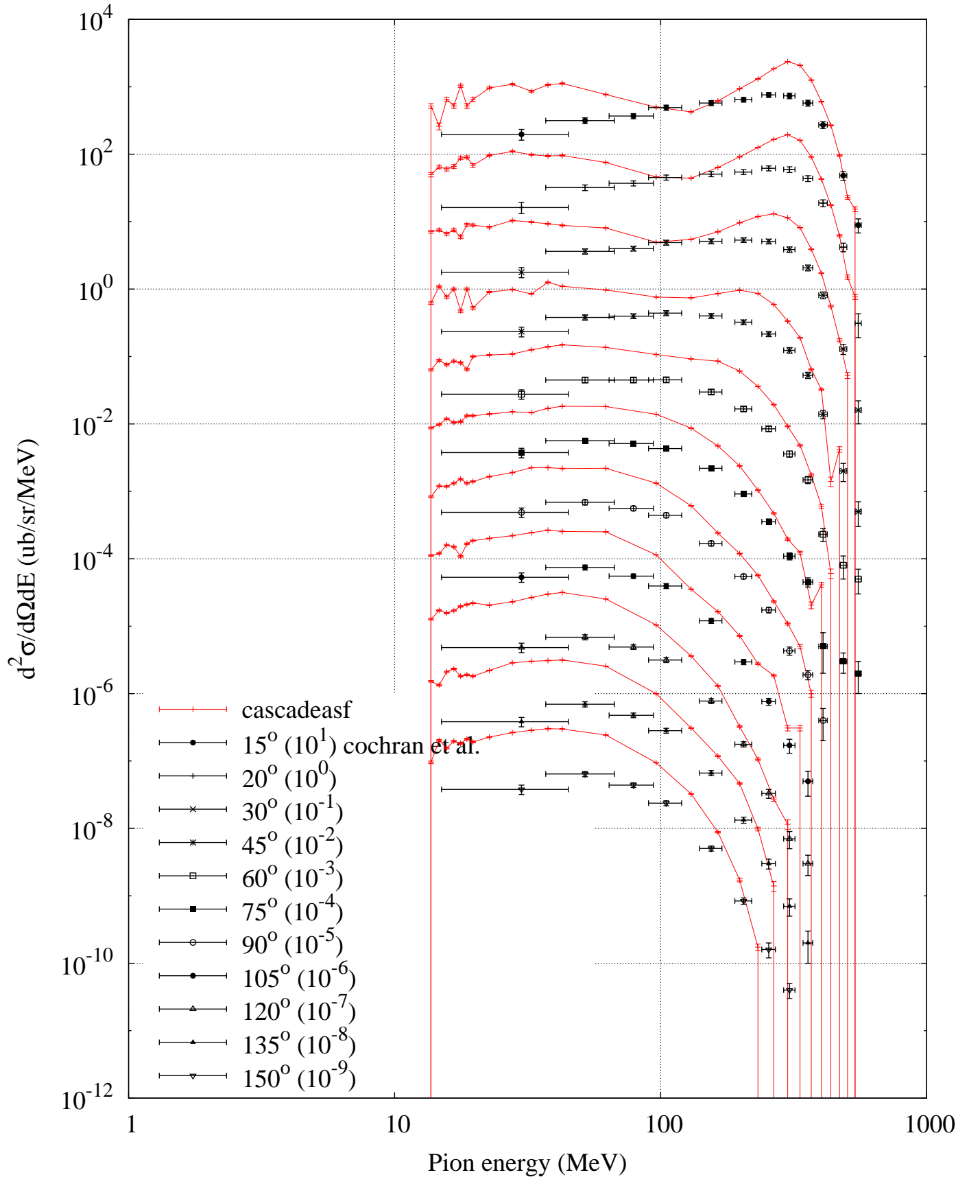
p (730 MeV) + Pb -- Pion plus spectrum
