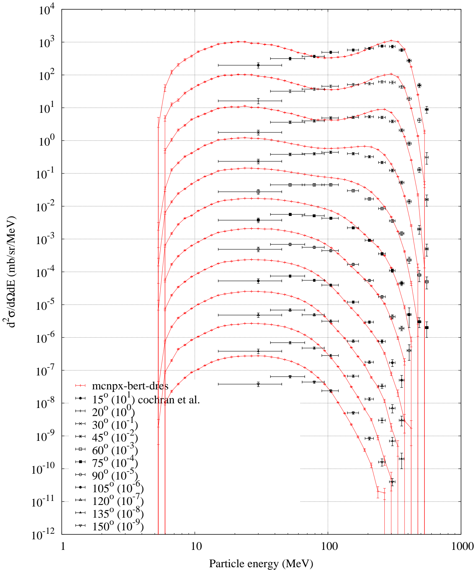
p (730 MeV) + Pb -- Pion plus spectrum
