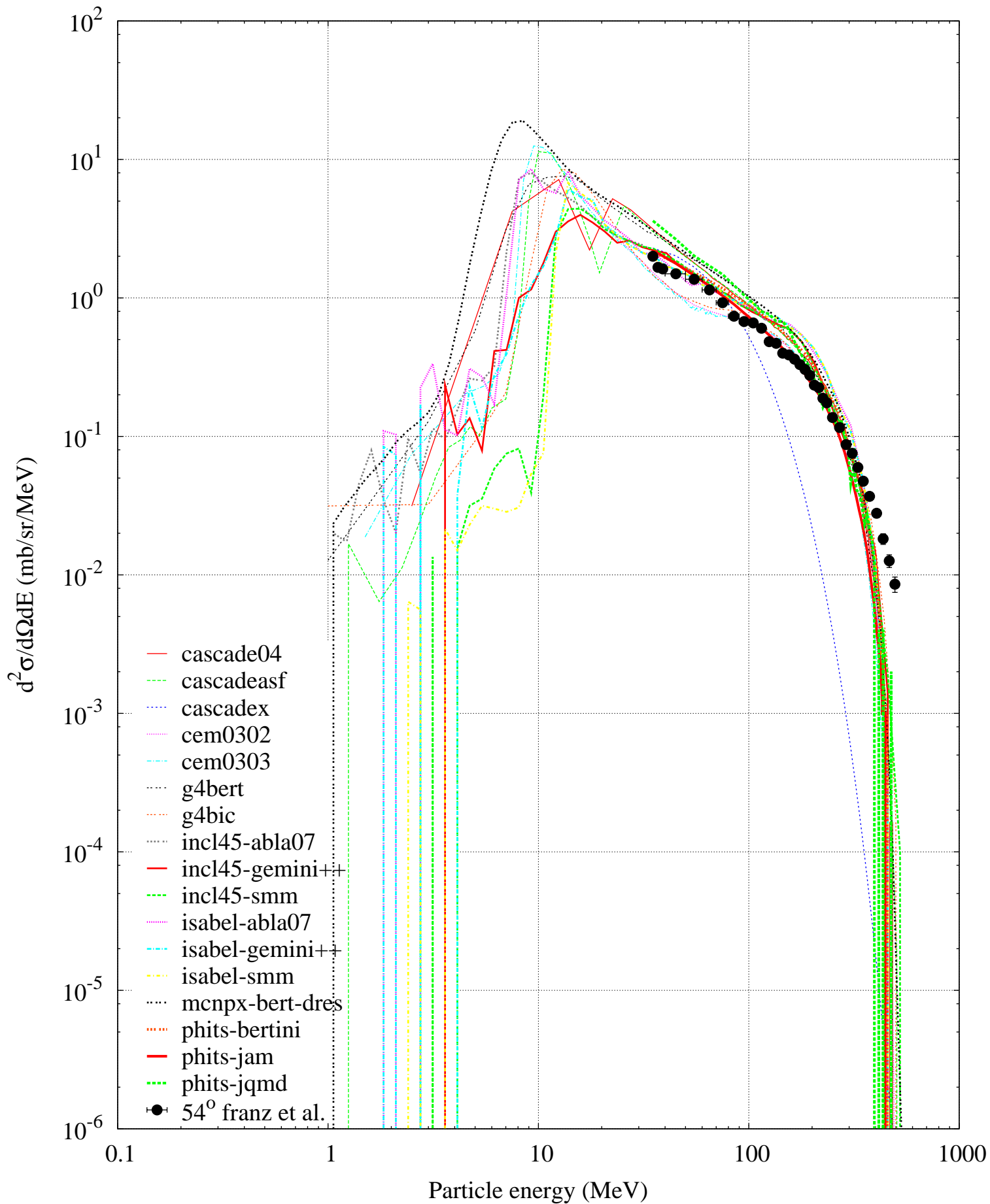
n (542 MeV) + Bi -- Proton spectrum
