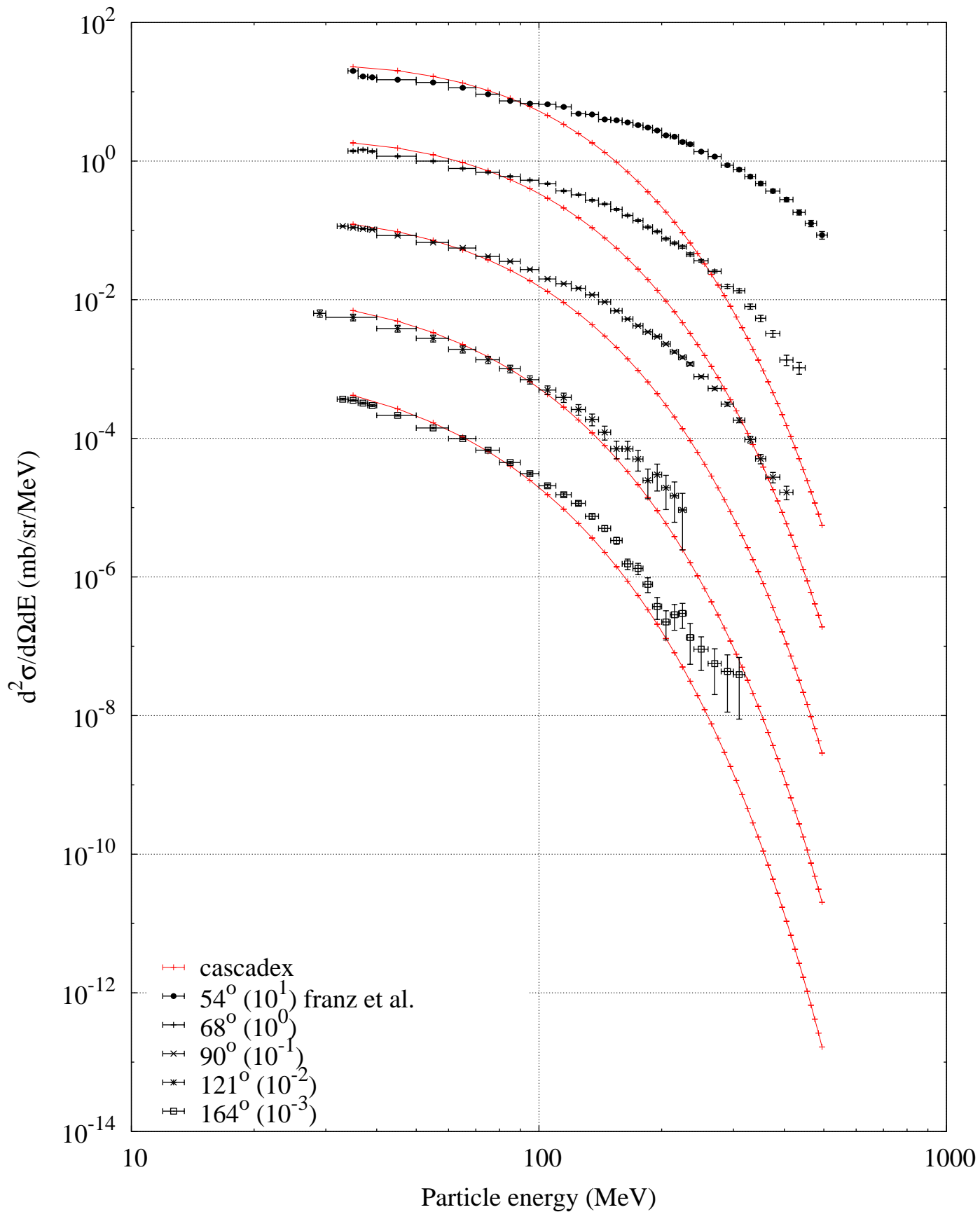
n (542 MeV) + Bi -- Particle spectrum
