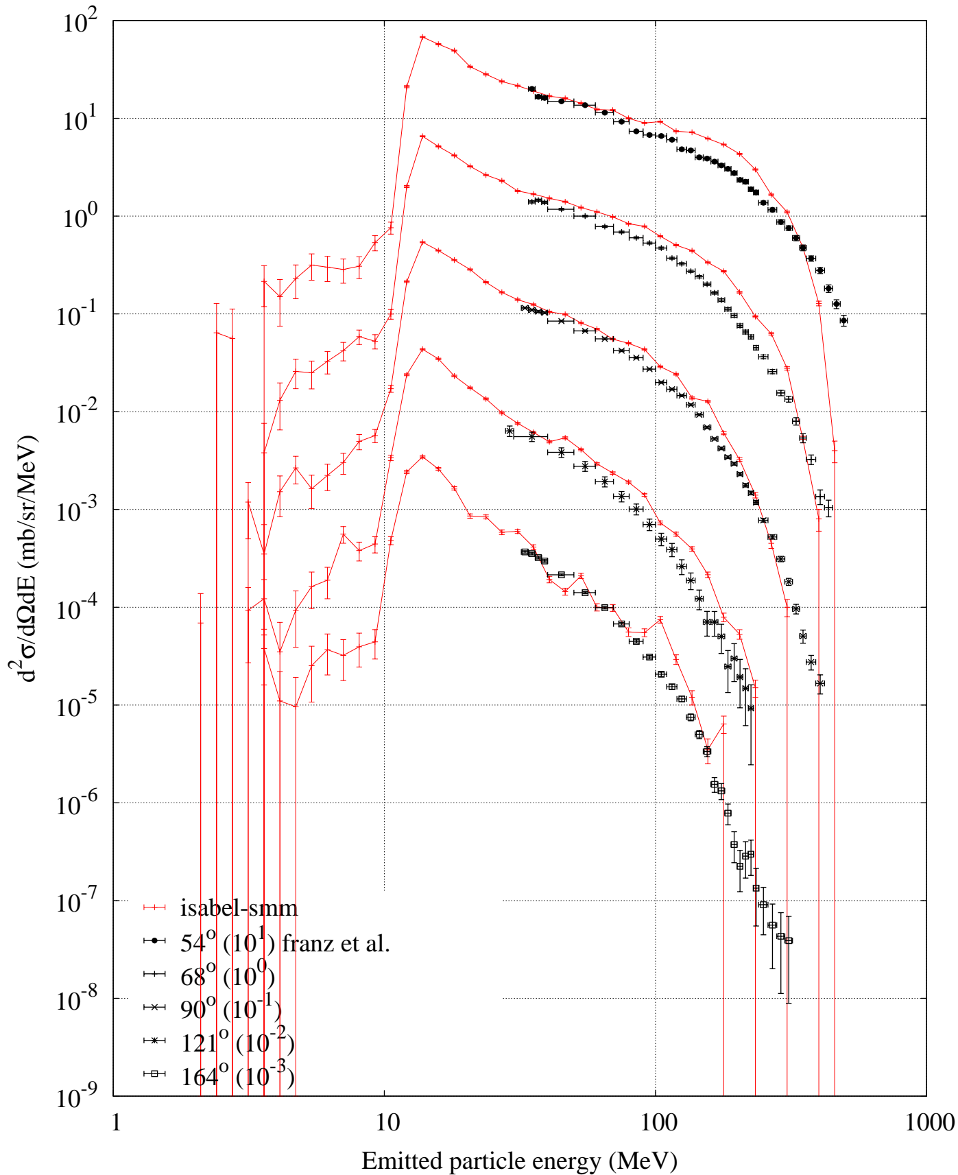
n (542 MeV) + Bi -- Proton spectrum
