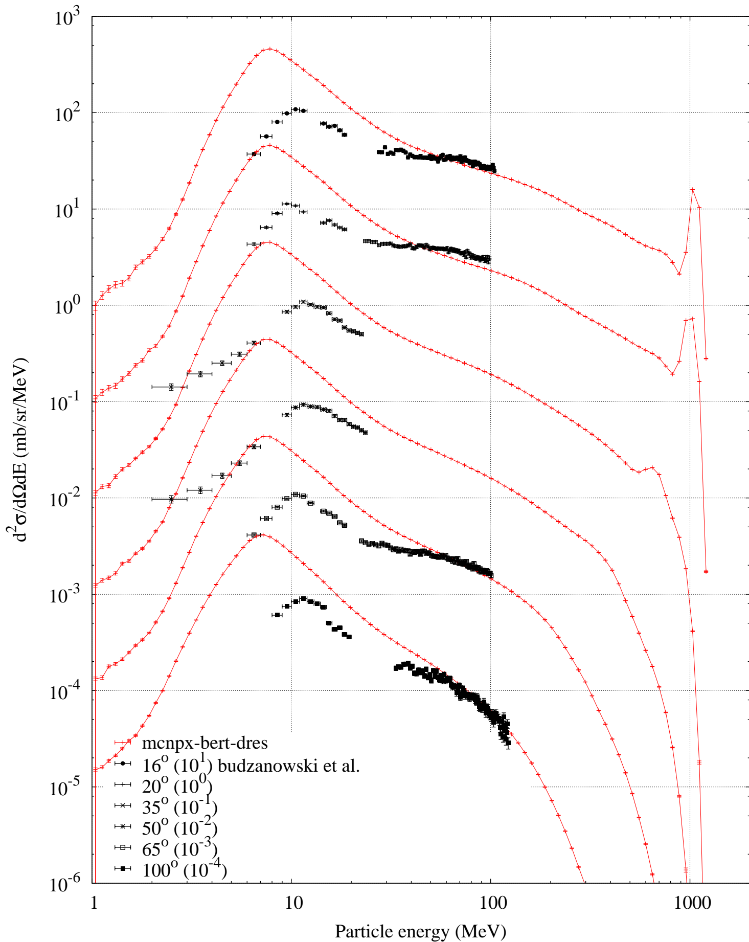
p (1200 MeV) + Au -- Proton spectrum
