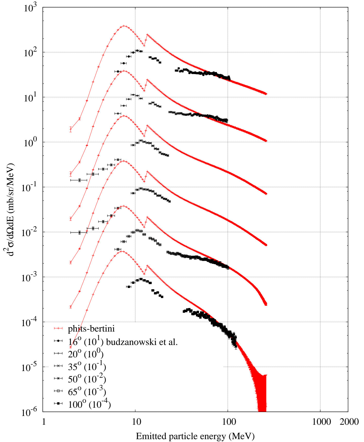
p (1200 MeV) + Au -- Proton spectrum
