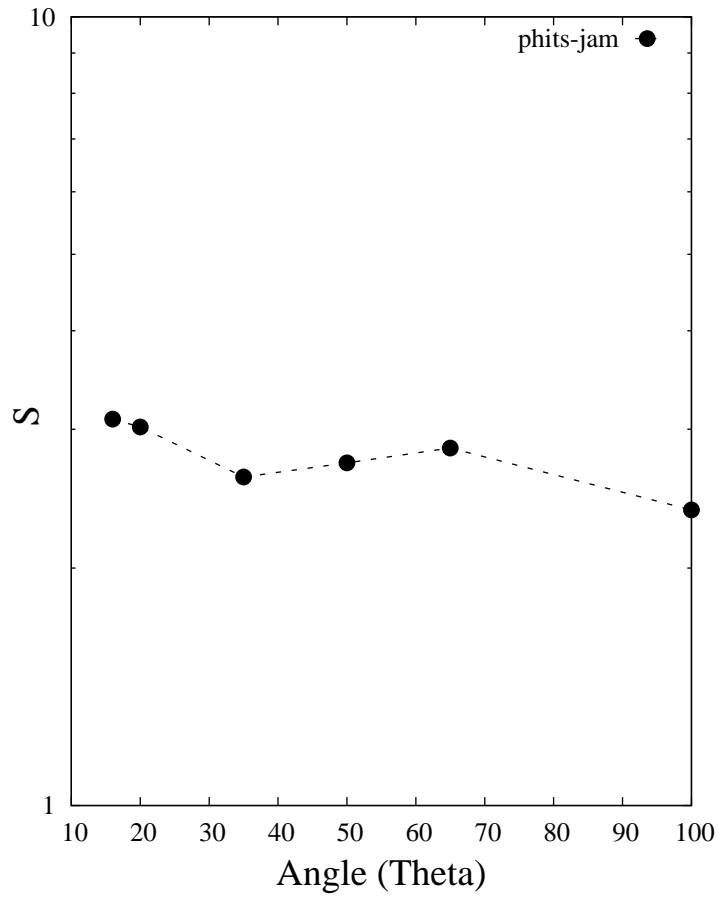
S factor - E_{\text{low}} (0-20 MeV)
