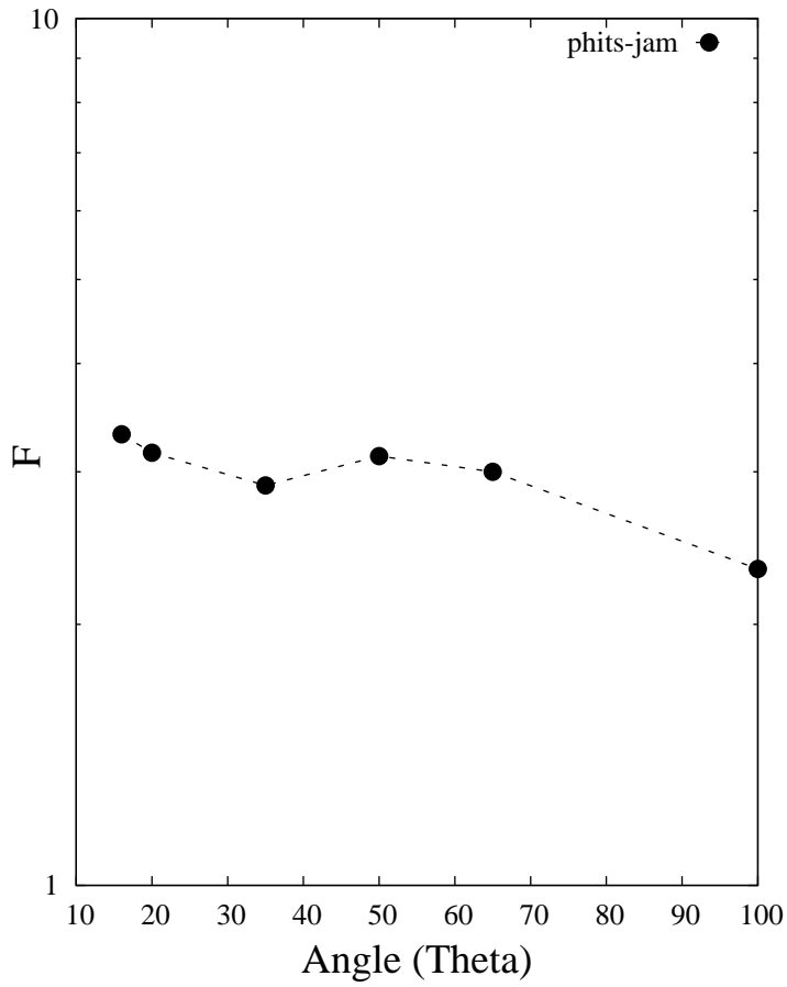
F factor - E_{\text{low}} (0-20 MeV)
