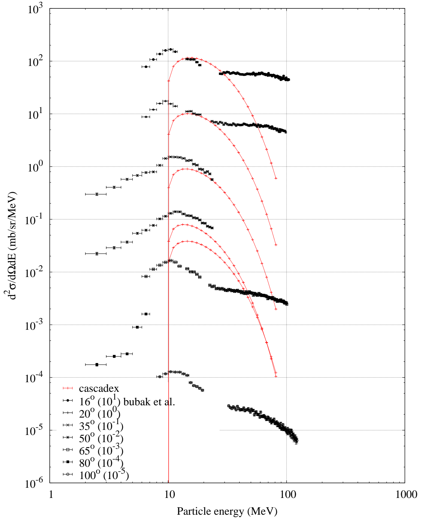
p (2500 MeV) + Au -- Particle spectrum
