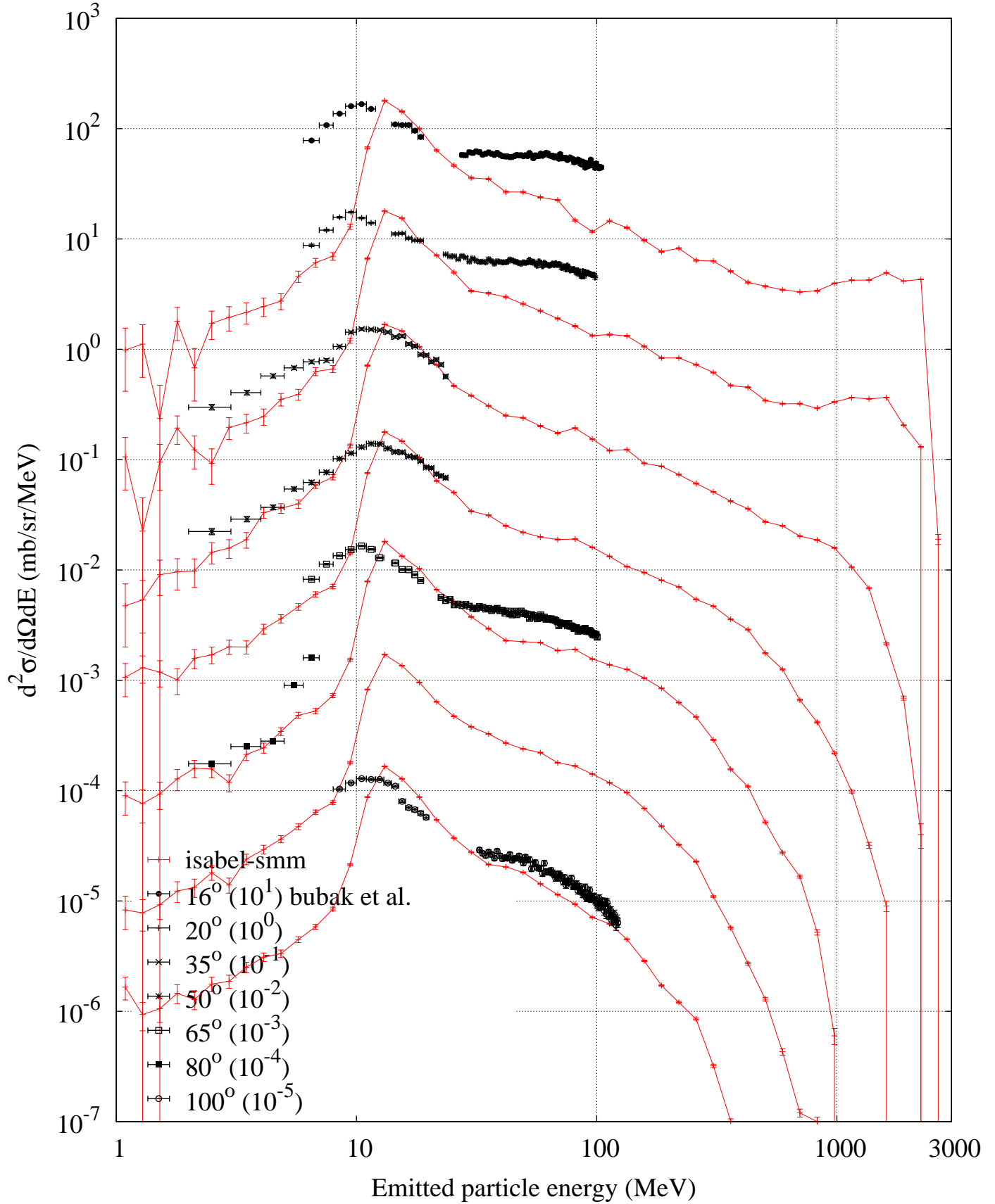
p (2500 MeV) + Au -- Proton spectrum
