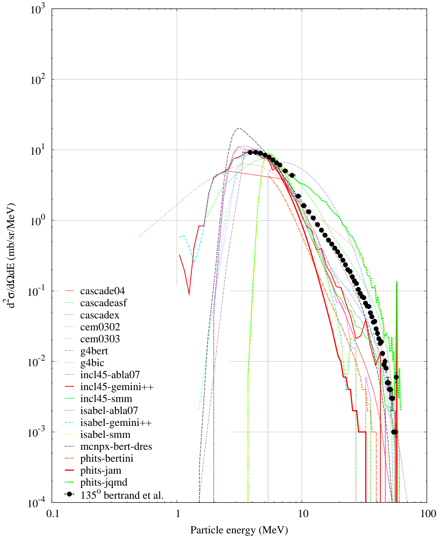
p (62 MeV) + Fe56 -- Proton spectrum
