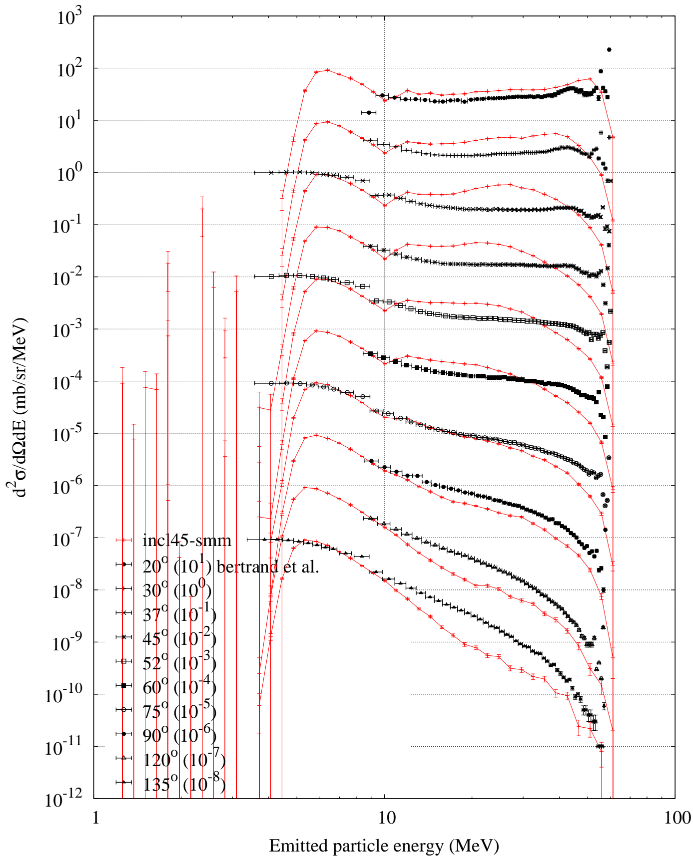
p (62 MeV) + Fe56 -- Proton spectrum
