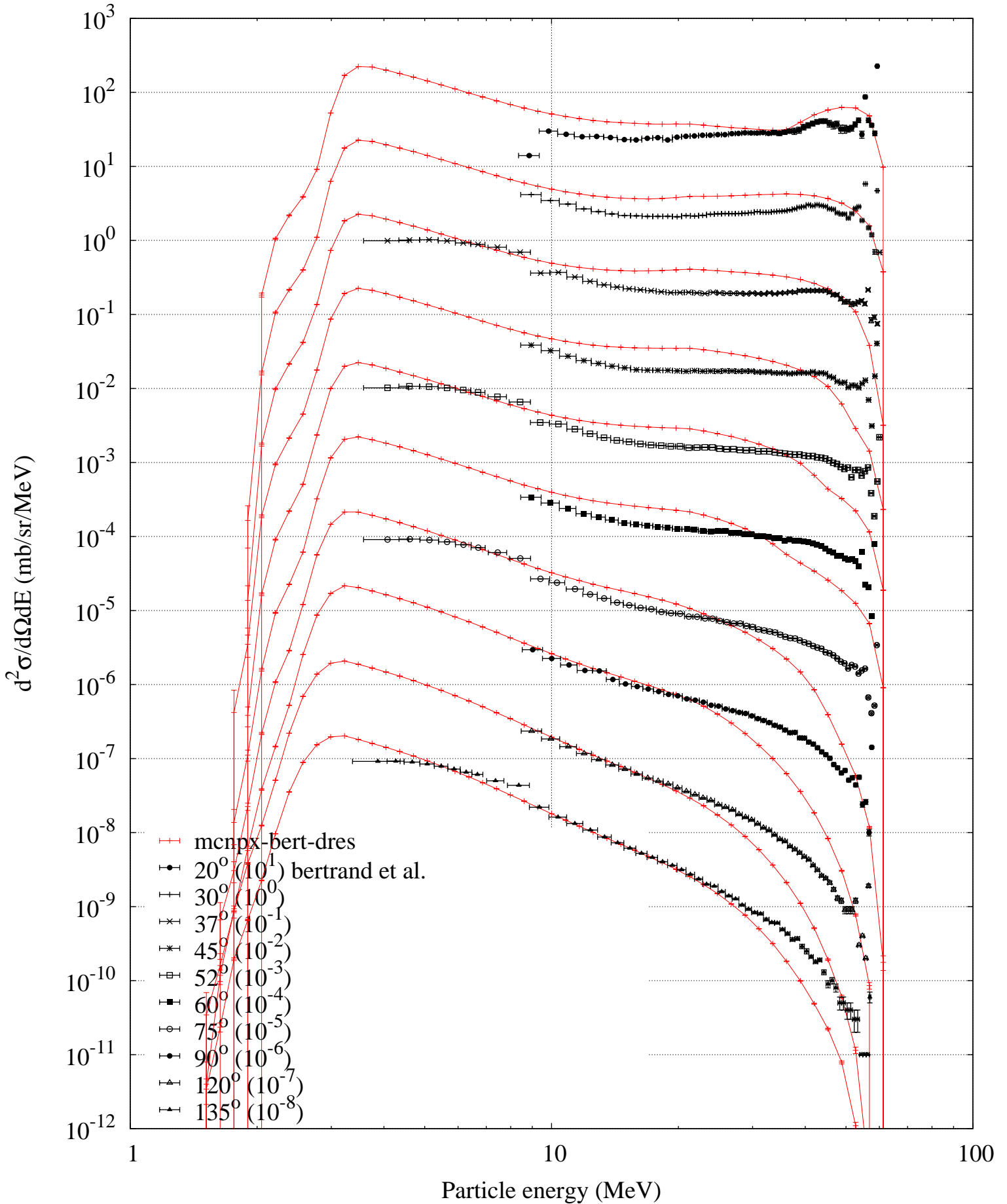
p (62 MeV) + Fe56 -- Proton spectrum
