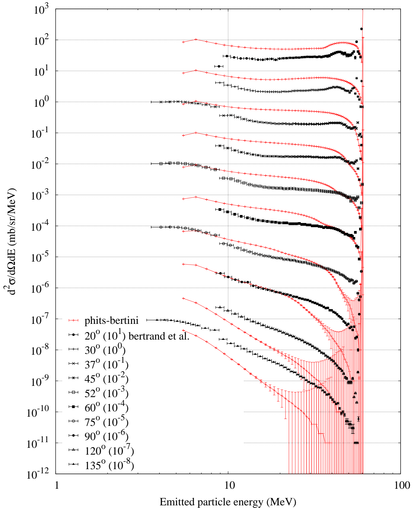
p (62 MeV) + Fe56 -- Proton spectrum
