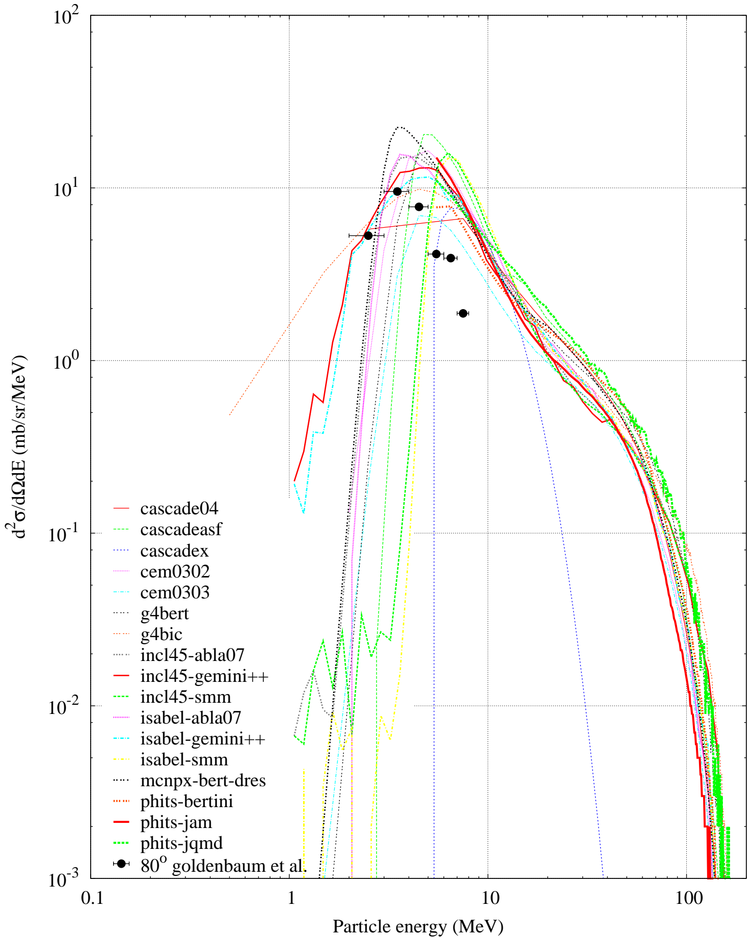
p (175 MeV) + Ni -- Proton spectrum
