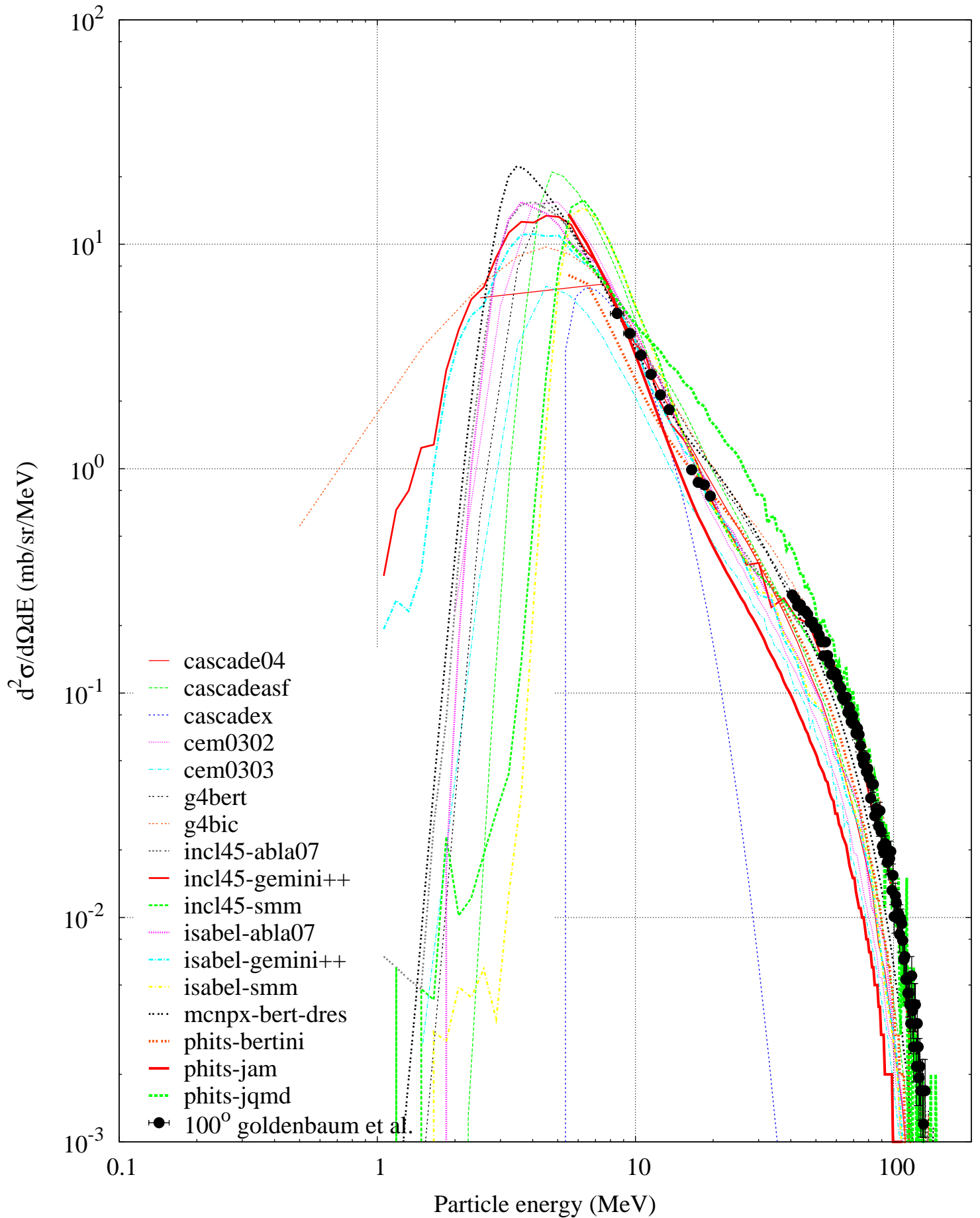
p (175 MeV) + Ni -- Proton spectrum
