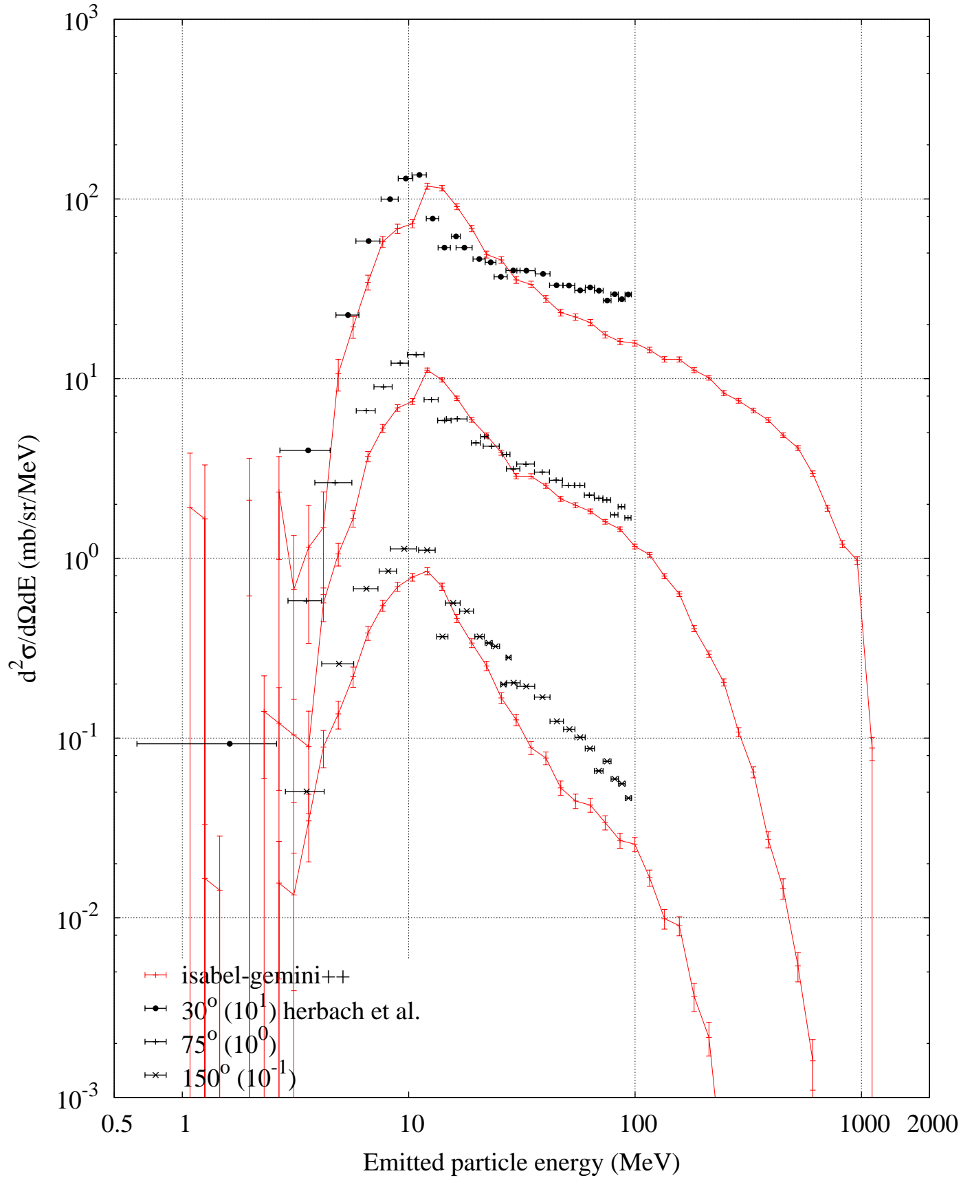
p (1200 MeV) + Ta -- Proton spectrum
