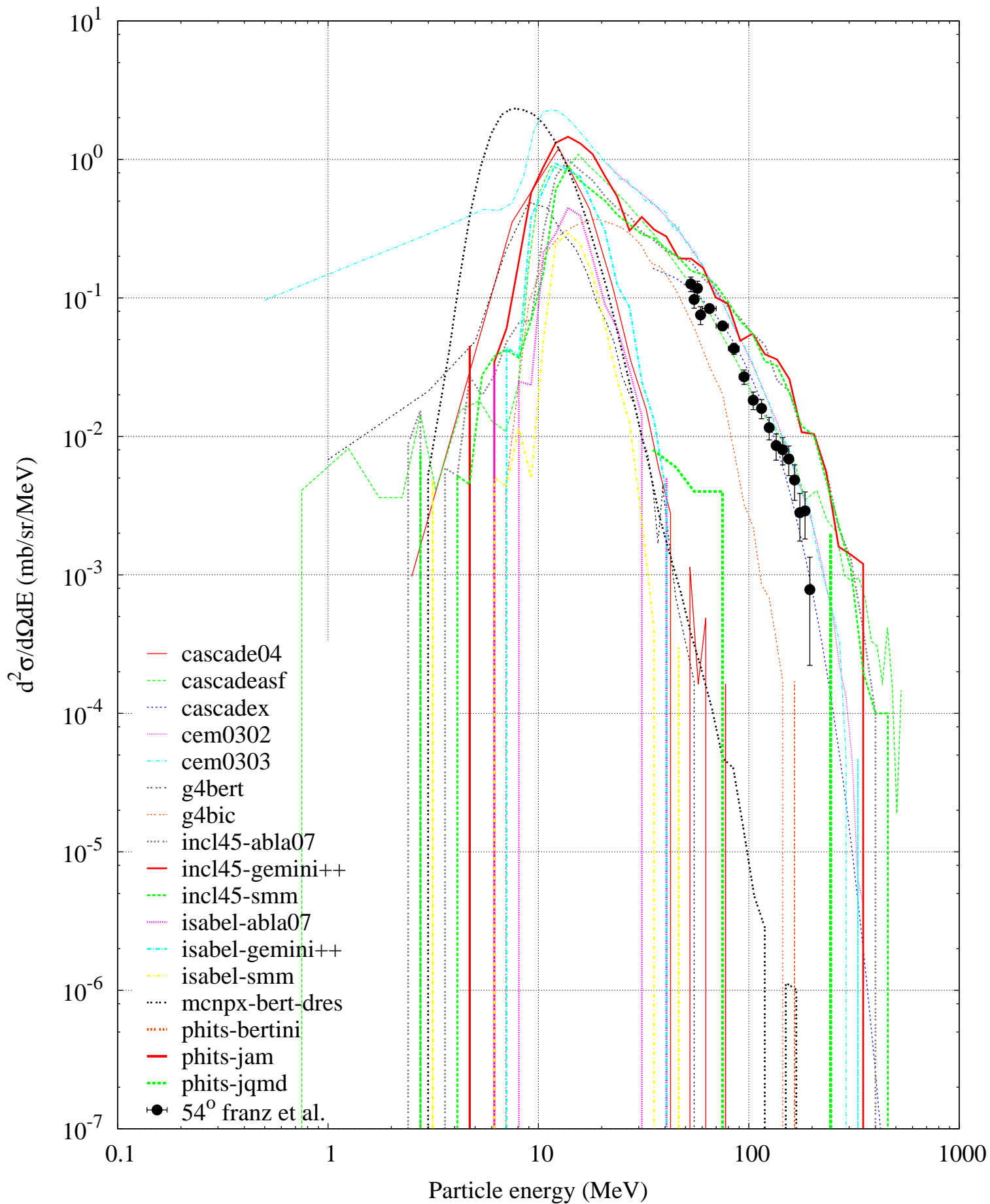
n (542 MeV) + Bi -- Triton spectrum
